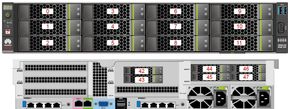
图 2-16 12x3.5 英寸硬盘直通配置
