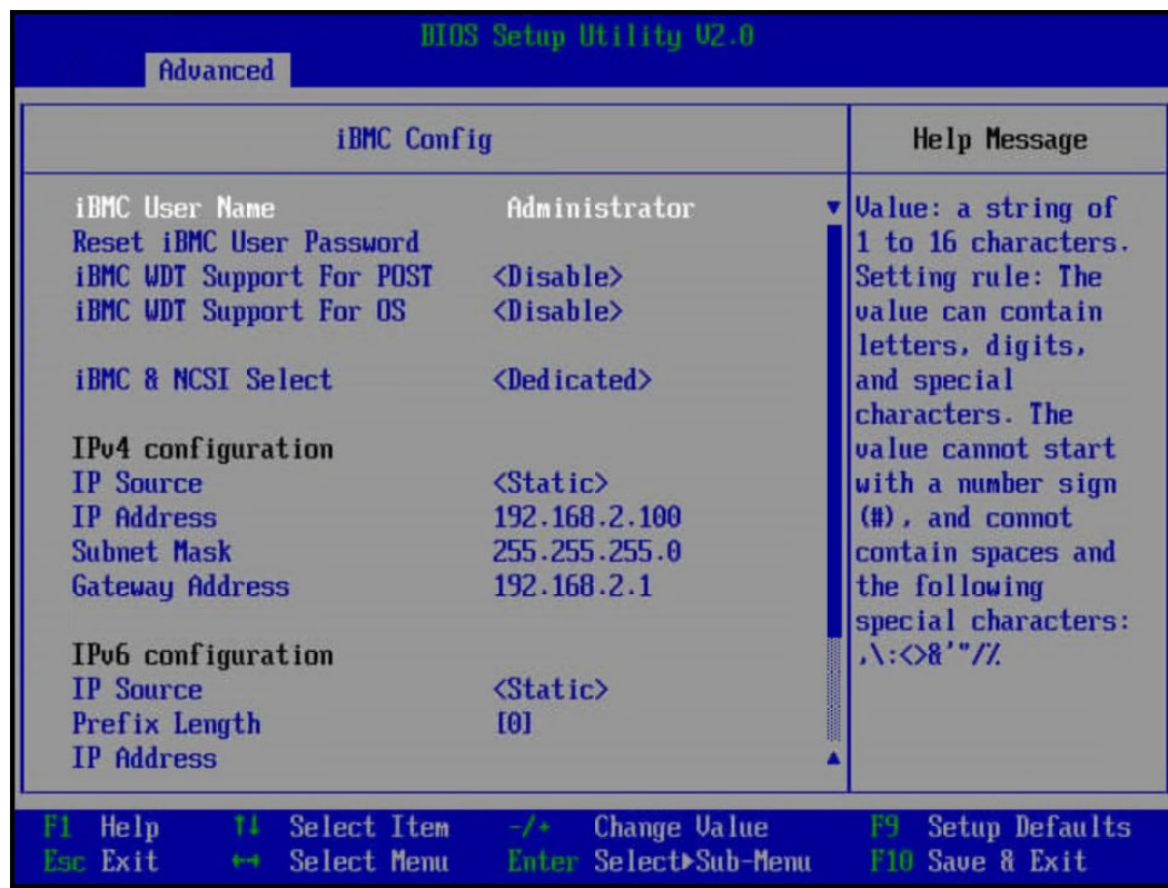
图 5-22 iBMC Config 界面 1
