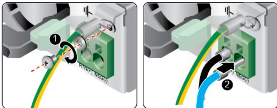
图 5-19 连接电源线缆（非 2000W 电源模块）
