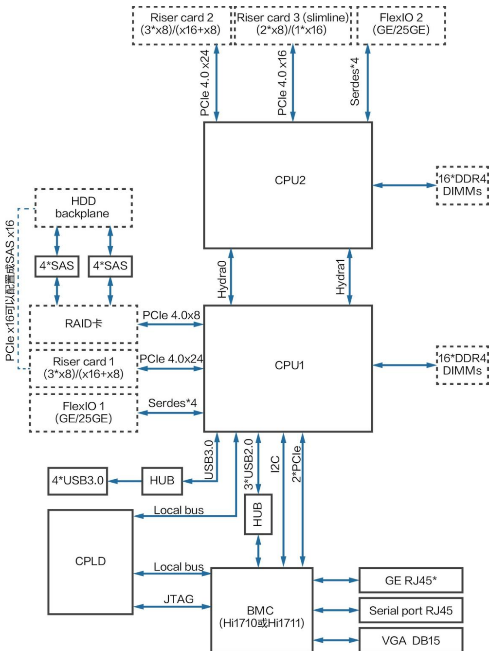
图 1-4 服务器逻辑结构（配置鲲鹏 920 7260 或 5250 处理器）
