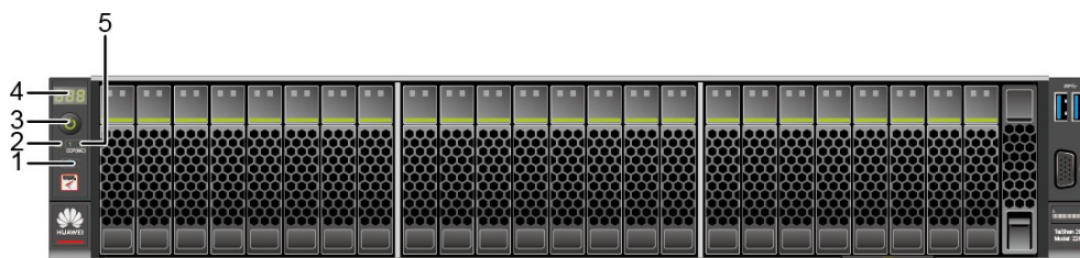
图 2-9 24x2.5 SAS/SATA 硬盘直通配置前面板指示灯和按钮
