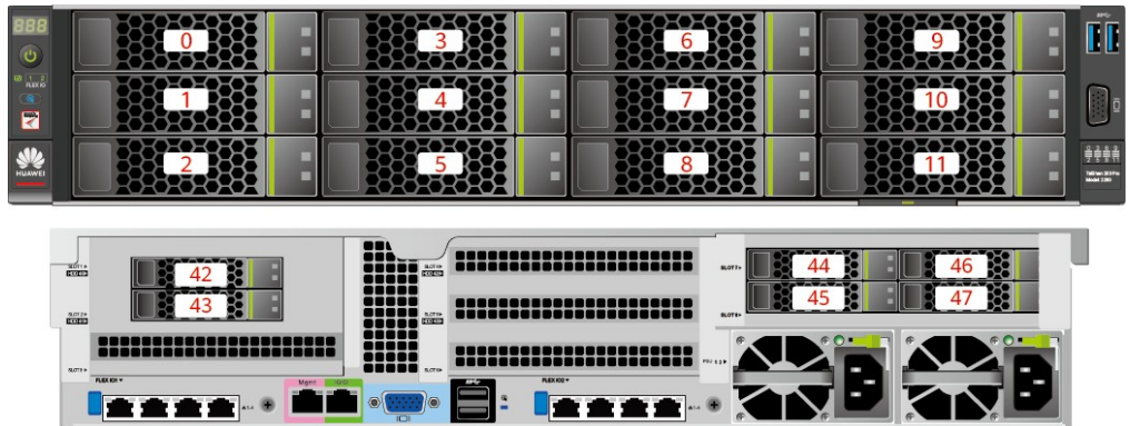
图 2-17 12x3.5 英寸硬盘 RAID 直通配置编号
