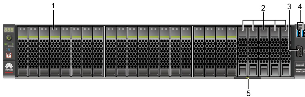
图 2-3 8x2.5 SAS/SATA+12x2.5 NVMe 硬盘配置前面板组件
