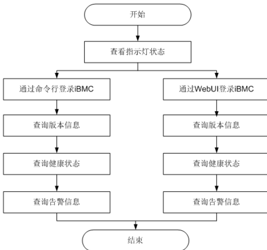
图 5-61 检查流程
