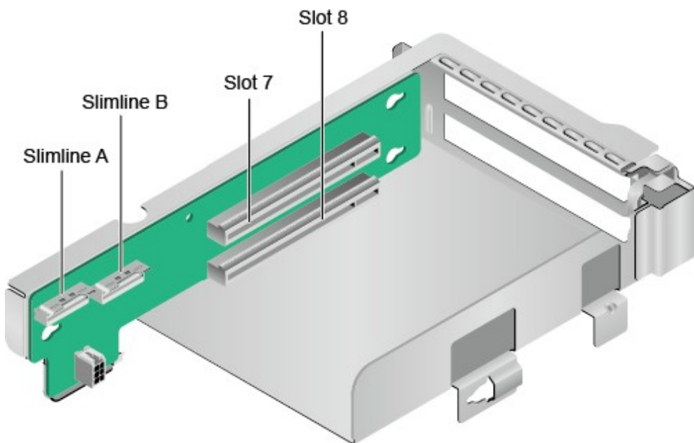
图 2-30 2x8 Riser 卡 6 (板名: BC82PRUF)
