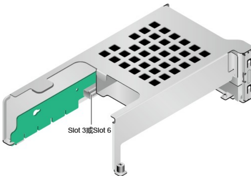
图 2-28 1x16 Riser 卡 4 (板名: BC82PRUC)
