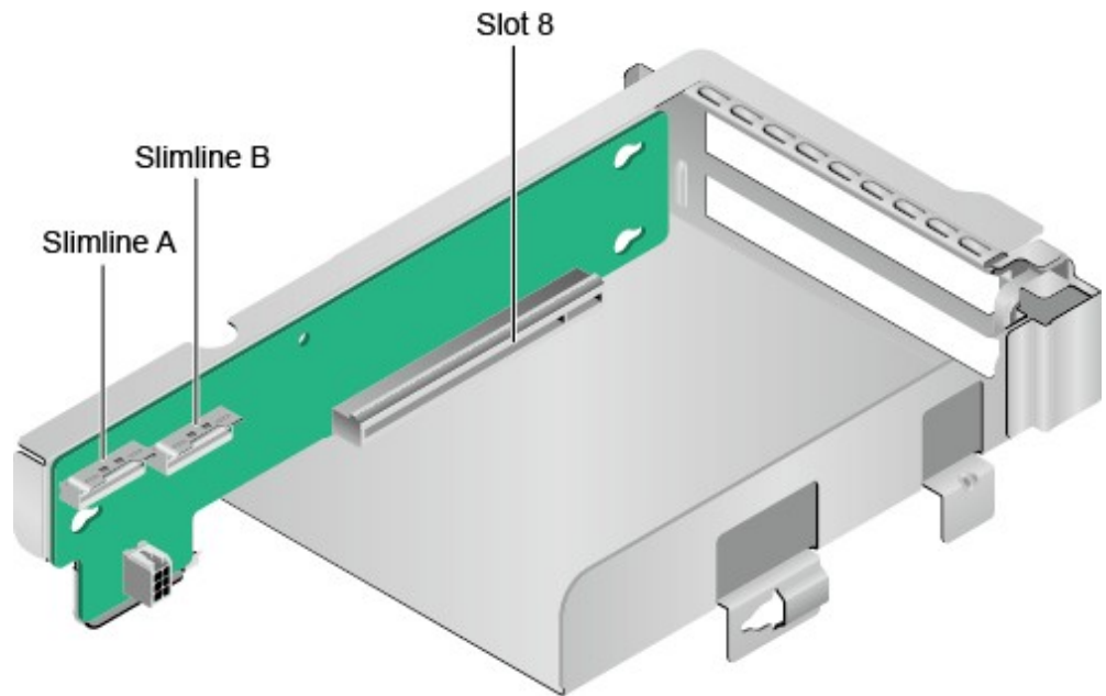
图 2-31 1x16 Riser 卡 7（板名：BC82PRUG）
