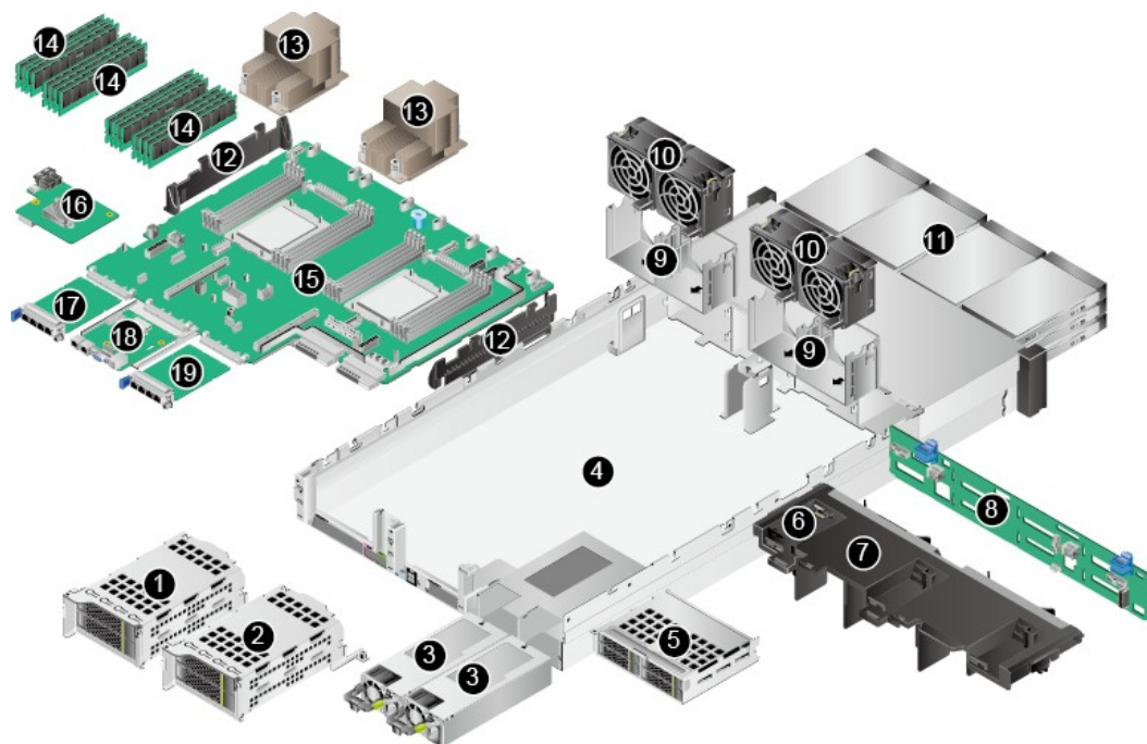
图 1-3 部件（配置鲲鹏 920 5220 或 3210 处理器）
