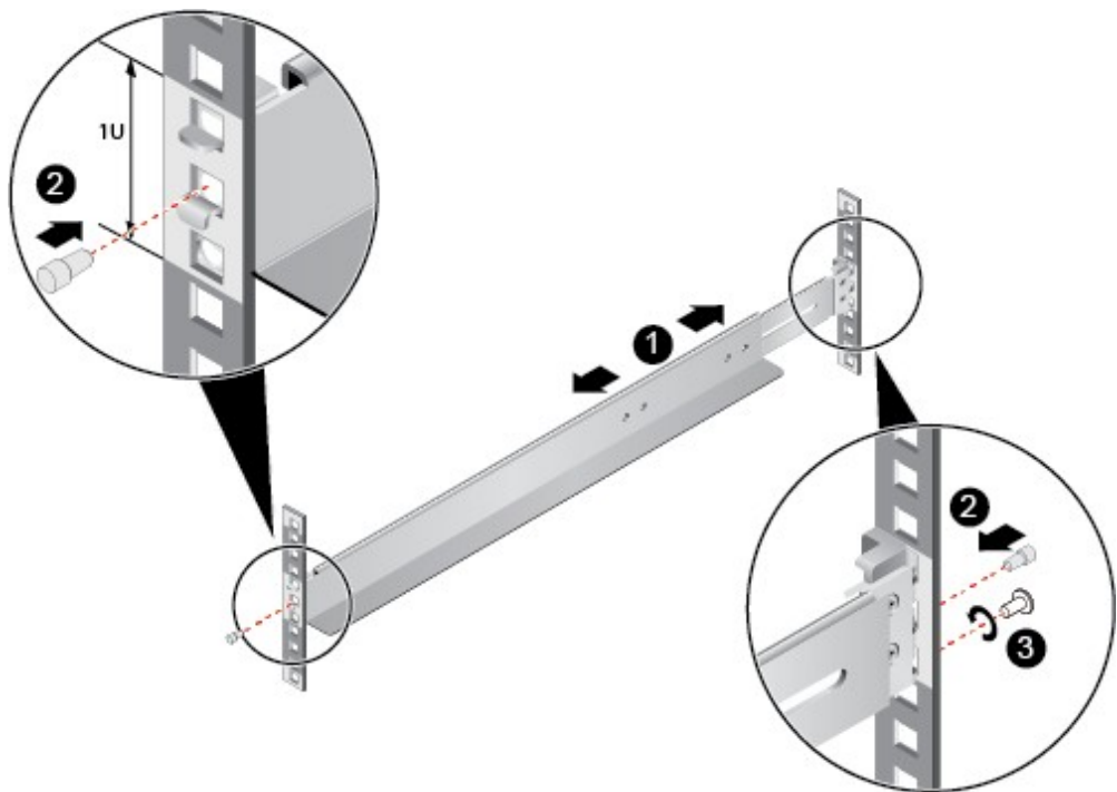
图 5-8 安装可伸缩滑道
