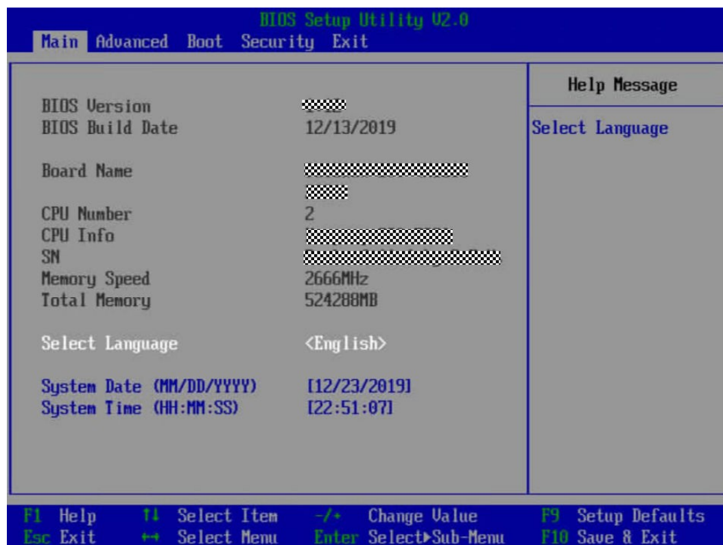
图 5-83 Main 界面
