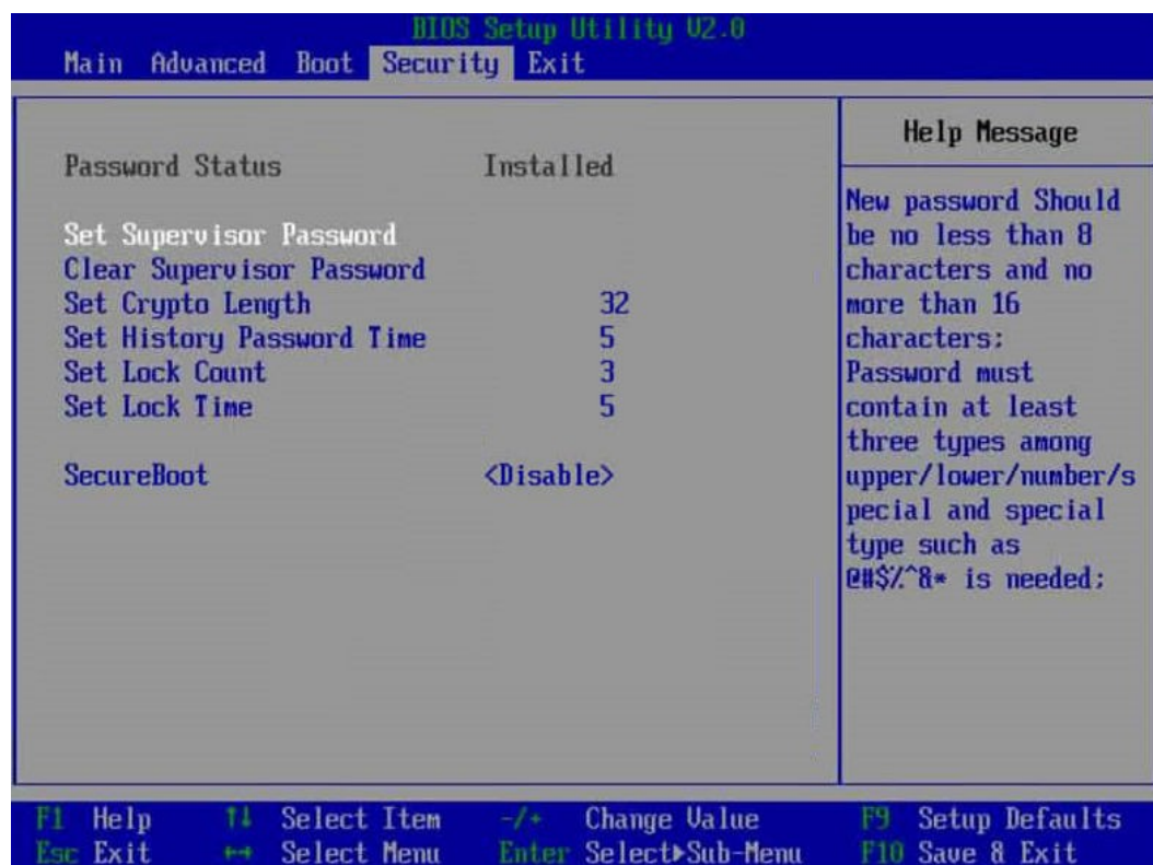
图 5-82 Security 界面
