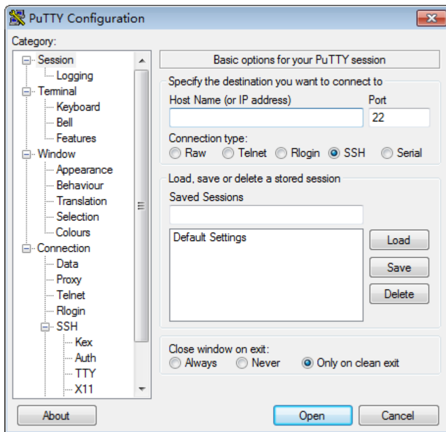
图 9-7 PuTTY Configuration
