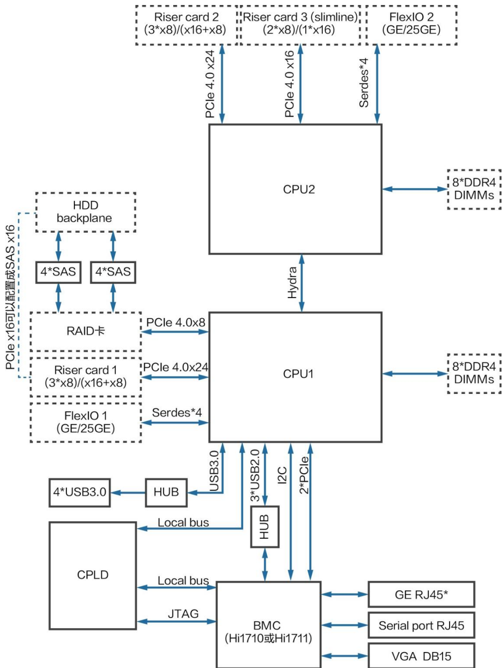
图 1-5 服务器逻辑结构（配置鲲鹏 920 5220 或 3210 处理器）
