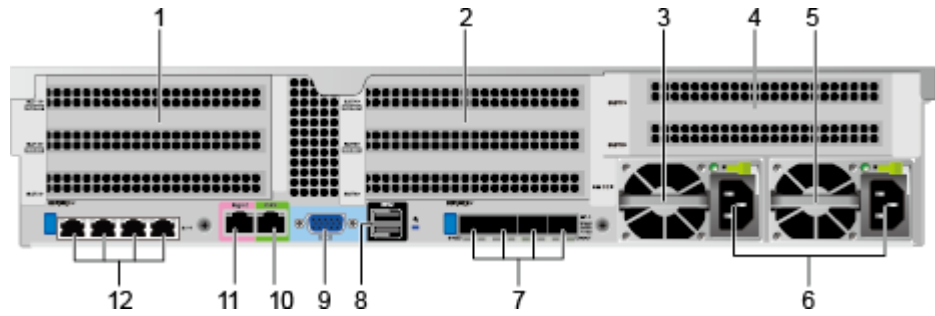
图 2-11 后面板组件
