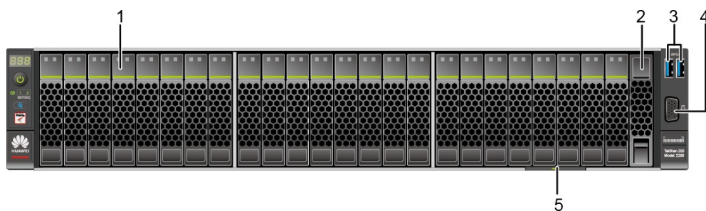
图 2-4 24x2.5 SAS/SATA 硬盘直通配置前面板组件
