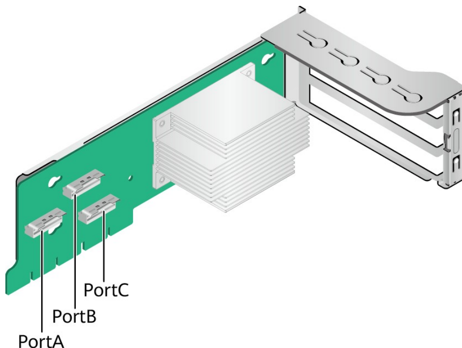
图 2-27 12NVMe 专用 Riser 卡 3 (板名: BC13PRTJA)
