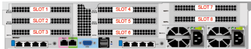
2-32 PCIe 插槽
