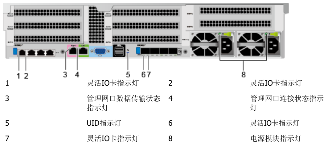
图2-12 后面板指示灯
