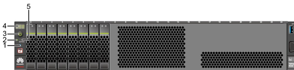
图 2-10 8x2.5 英寸硬盘配置前面板指示灯和按钮
