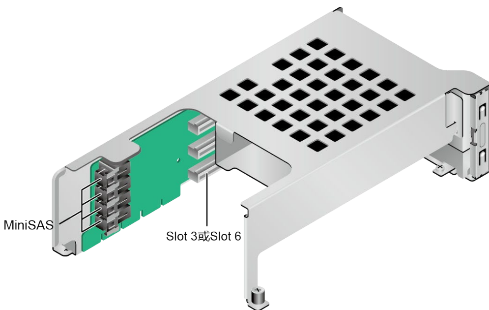
图 2-29 SAS Riser 卡 5 (板名: BC82PRNE)
