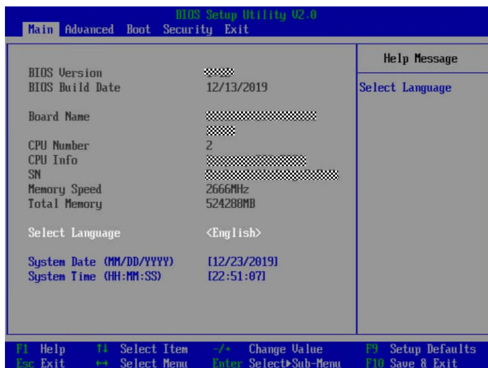
图 5-45 Main 界面
