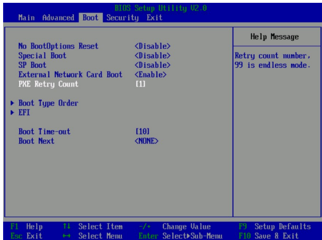
图 5-74 Boot 界面
