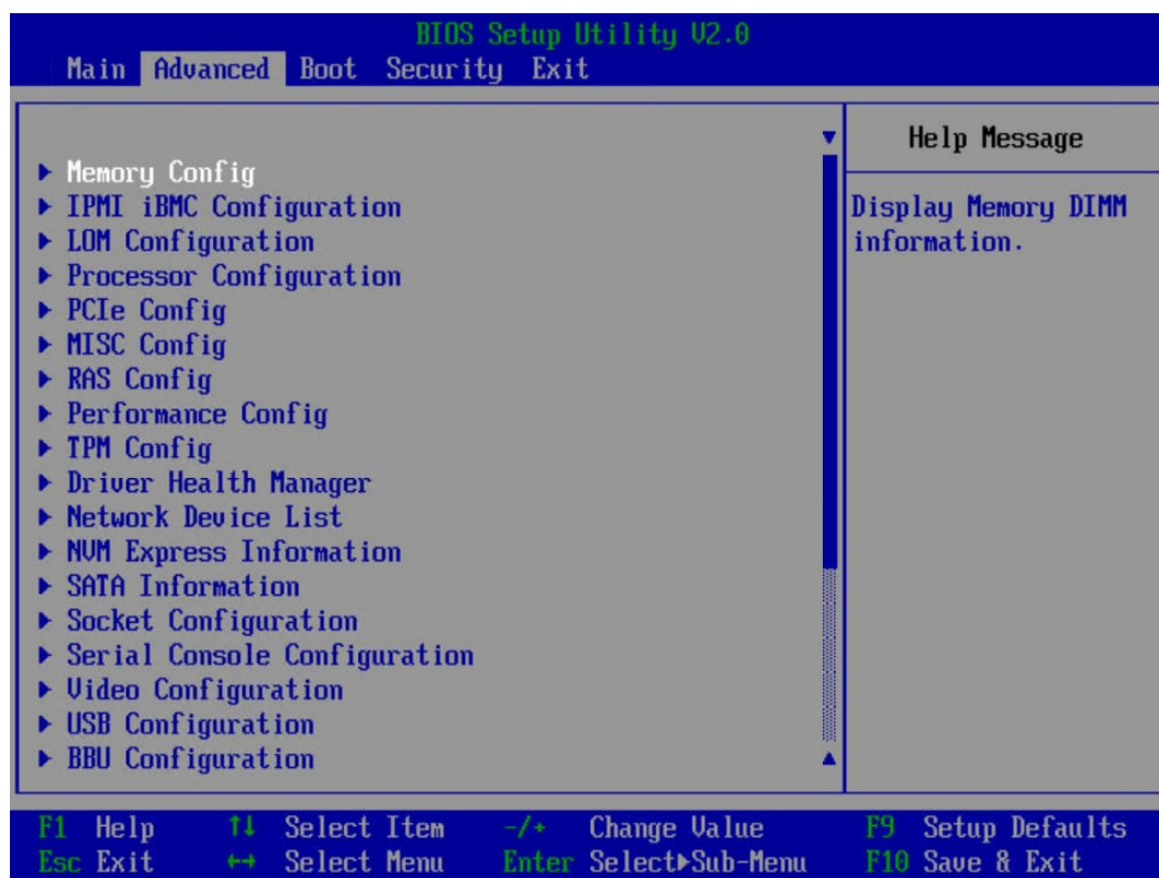
图 5-78 Advanced 界面
