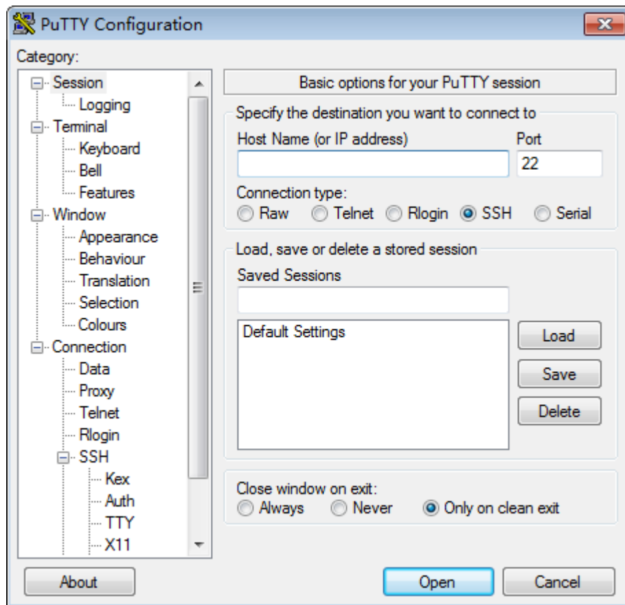
图 8-10 PuTTY Configuration
