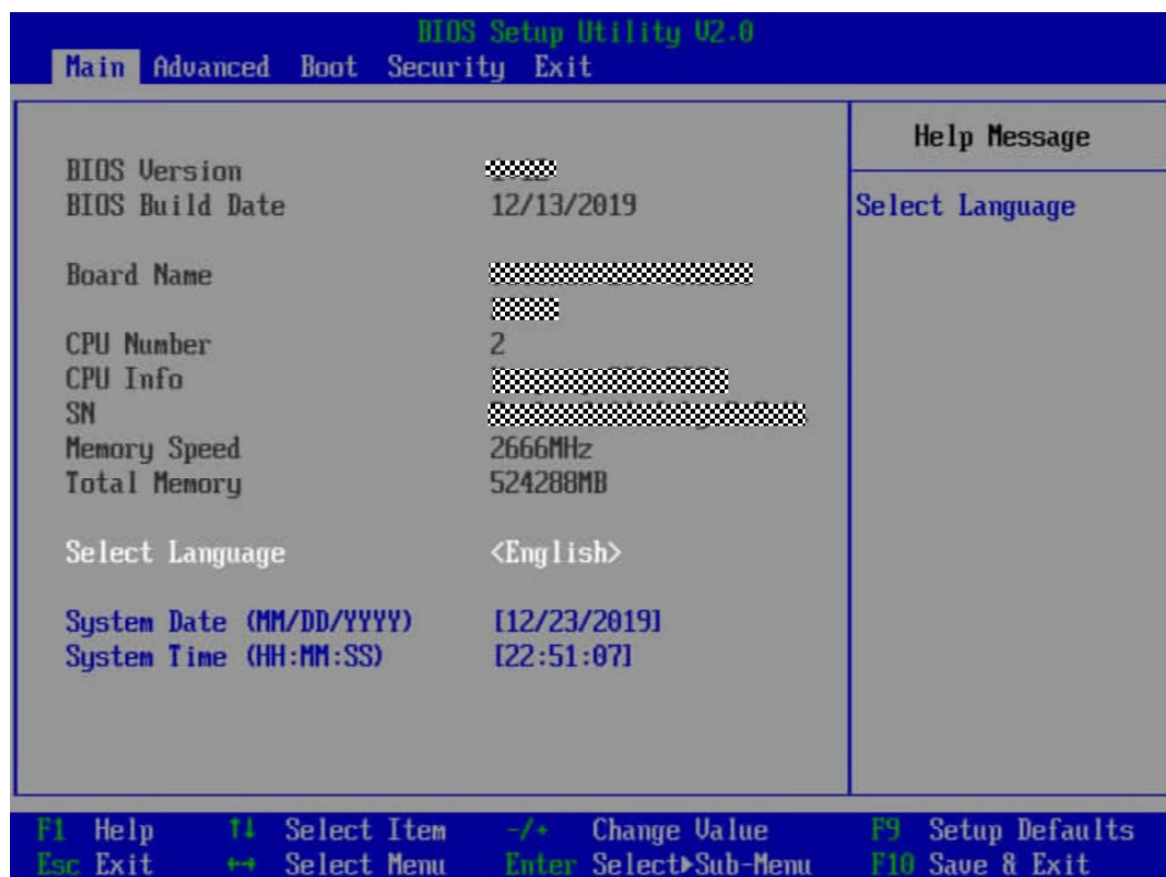
图 5-55 Main 界面
