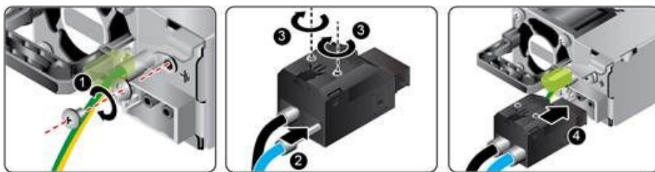
图 5-20 连接电源线缆（2000W 电源模块）
