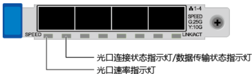
图 2-14 TM280（4x25GE 光口）
