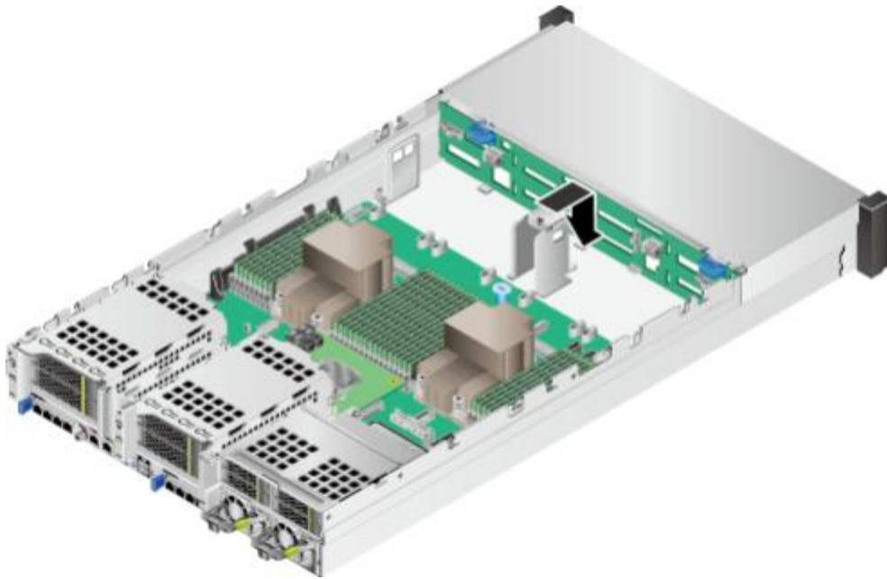
图 5-82 安装硬盘背板
