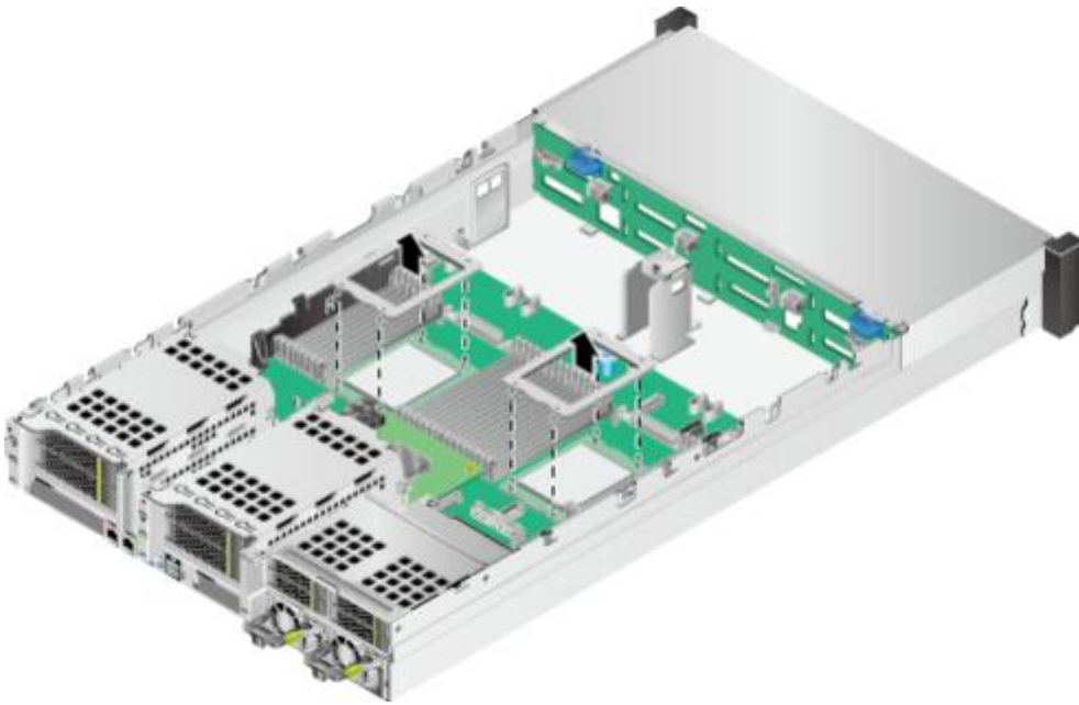
图 5-99 拆卸 CPU 散热器托架
