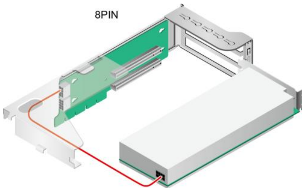
图 5-60 连接 GPU 显卡电源线缆
