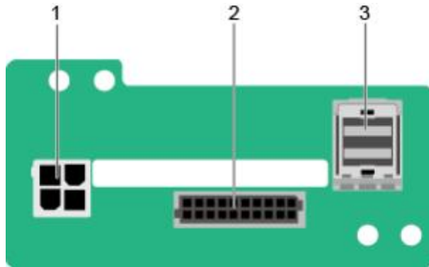
图 2-31 2x2.5 英寸后置硬盘背板( Part No.: 03025WCM )
