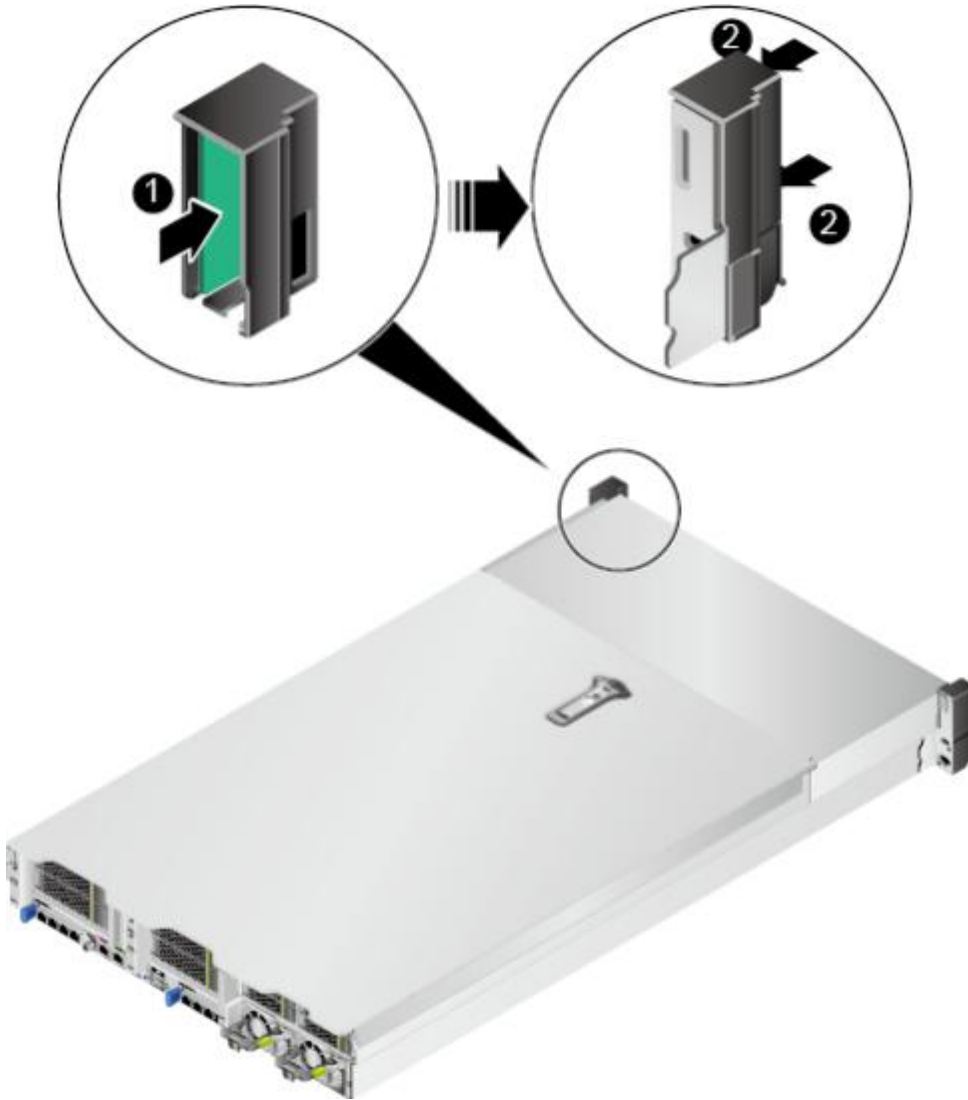
图 5-95 安装右挂耳板
