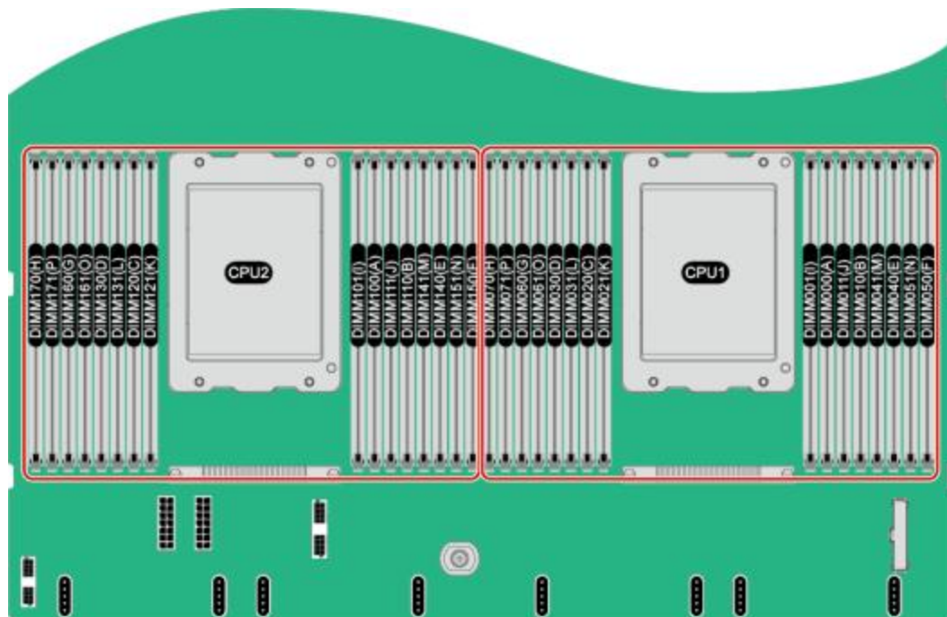
图 2-35 内存槽位编号(配置鲲鹏 920 7260 或 5250 处理器)
