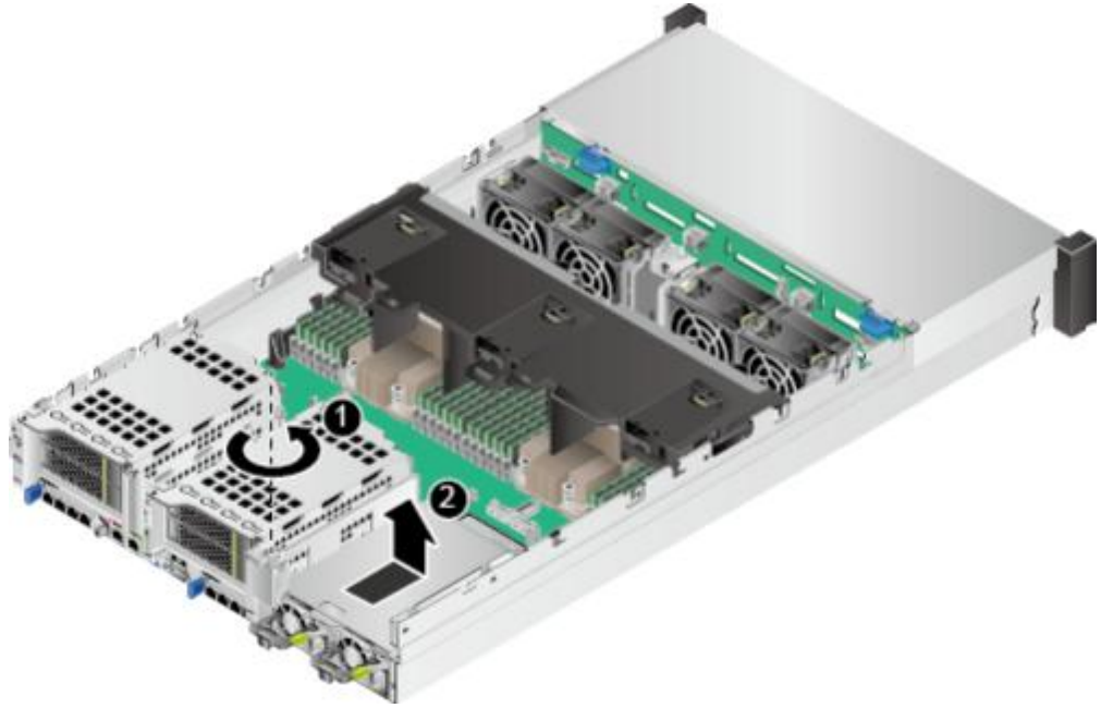
图 5-45 拆卸 Riser 模组 3 的下托架
