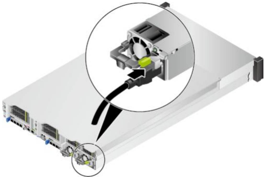
图 5-25 连接电源线缆
