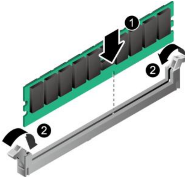
图 5-75 安装 DIMM
