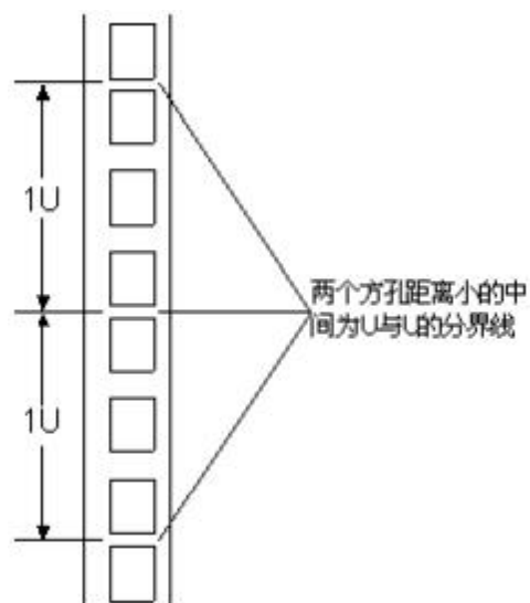
图 5-3 机柜导槽 U 与 U 的间距区分示意图
