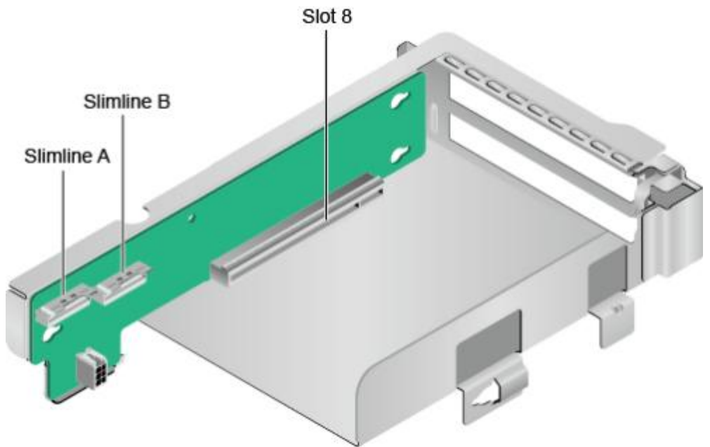
图 2-43 1x16 Riser 卡 7 (板名: BC82PRUG)
