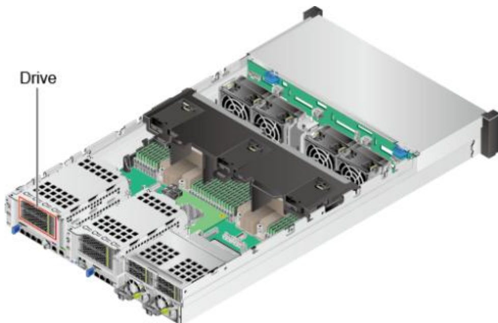
图 5-84 硬盘位置
