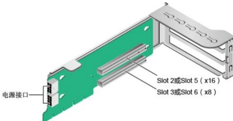
图 2-38 1x8+1x16 Riser 卡 2 (板名: BC82PRUB)
