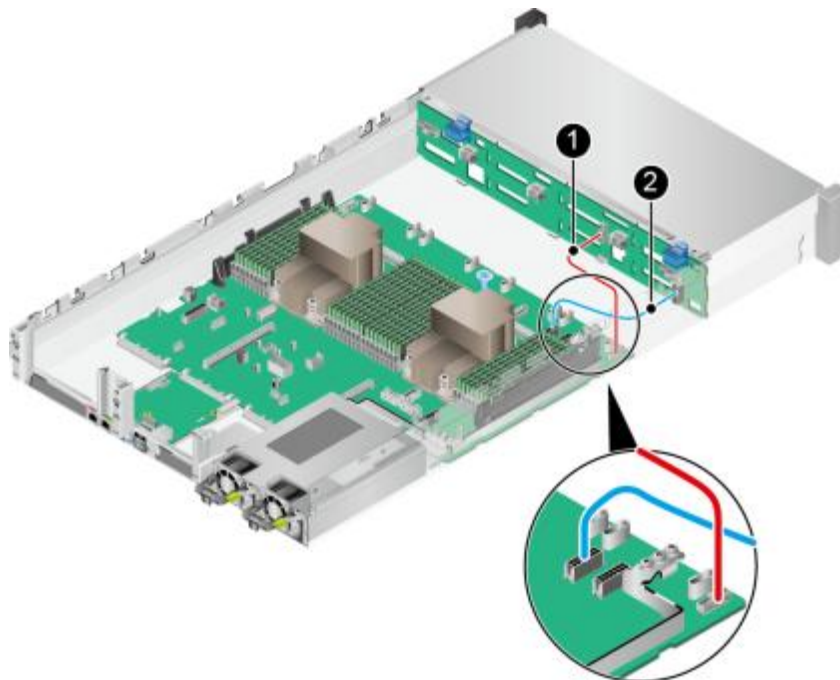
图 3-12 前置硬盘背板的电源线和低速信号线
