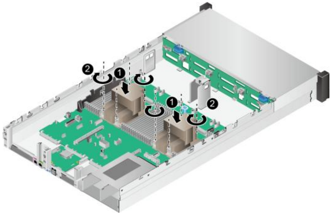
图 5-108 安装 CPU 散热器
