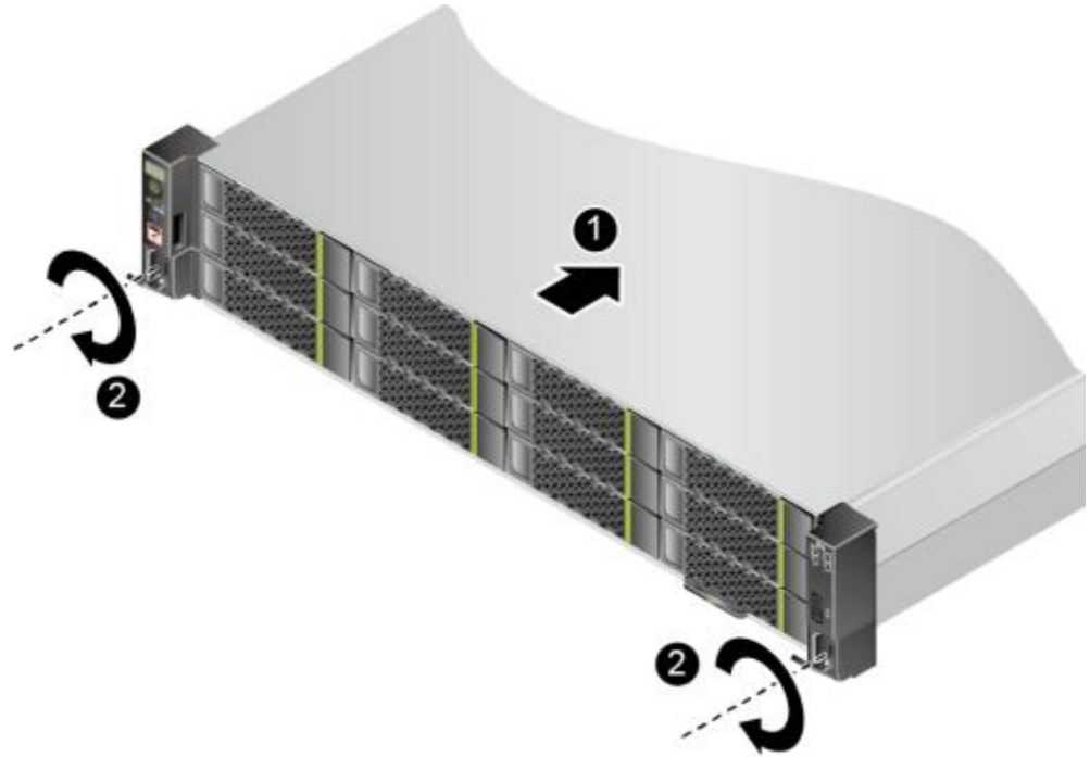
图 5-6 安装服务器
