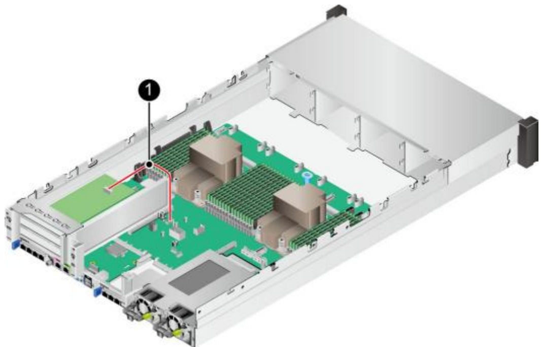
图 3-30 NC-SI 连线
