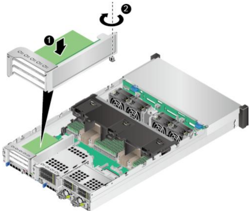
图 5-52 安装 Riser 模组 1
