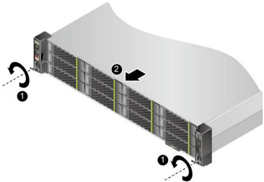
图 5-11 拆卸服务器
