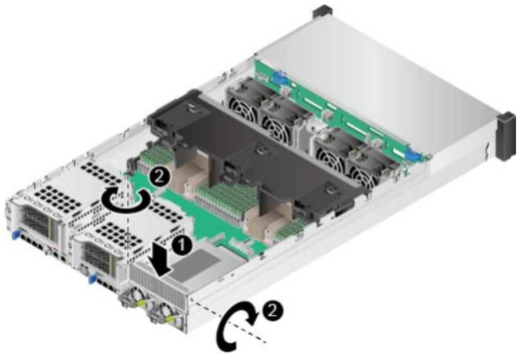
图 5-48 安装空闲挡板(3)
