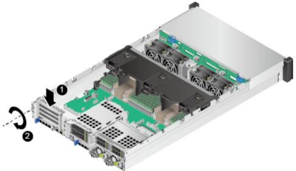
图 5-46 安装空闲挡板(1)
