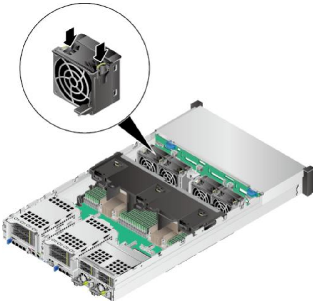
图 5-41 安装风扇模块
