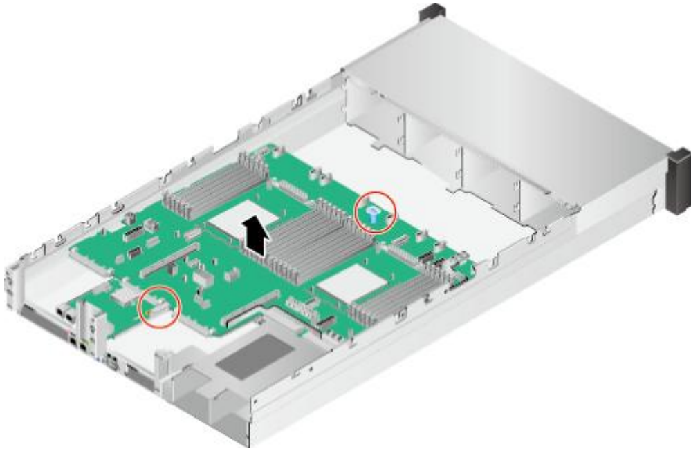
图 5-102 拆卸主板
