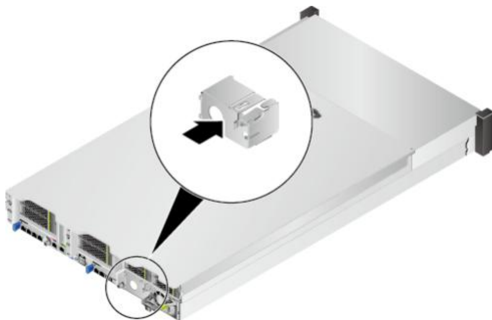
图 5-22 安装电源空闲挡板
