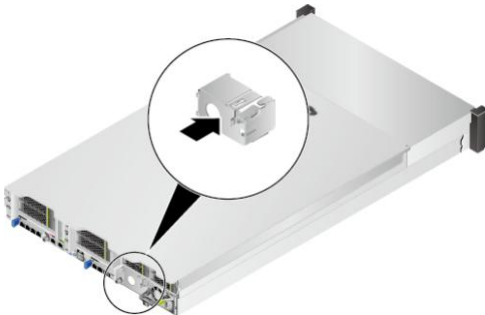
图 5-30 安装电源空闲挡板
