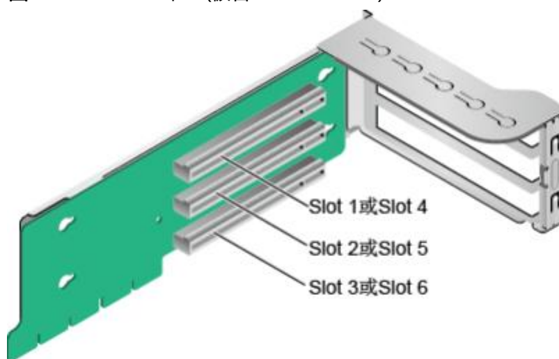
图 2-37 3x8 Riser 卡 1 (板名: BC82PRUA)
