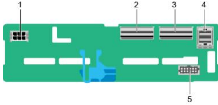
图 2-32 4x2.5 英寸后置硬盘背板( Part No.: 03025VYV)
