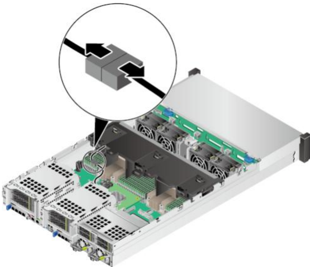
图 5-36 拆卸超级电容线缆
