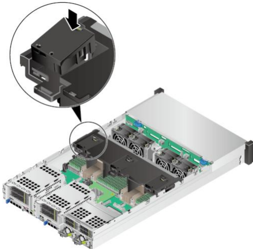
图 5-71 安装超级电容支架
