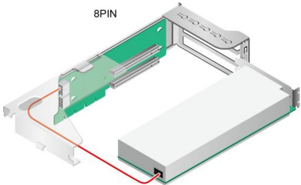
图 3-20 连接 GPU 卡电源线缆
