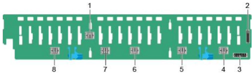
图 2-28 24x2.5 英寸硬盘背板( Part No.: 03026VRD)
