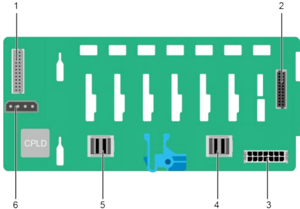
图 2-29 8x2.5 英寸硬盘背板( Part No.: 03026VRB)
