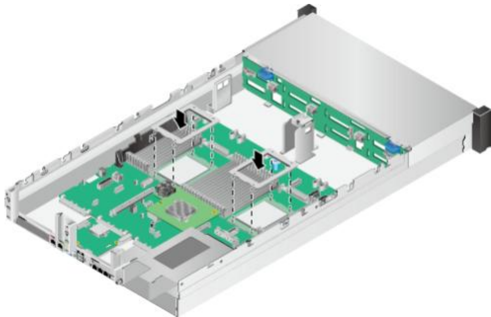
图 5-106 安装 CPU 散热器托架
