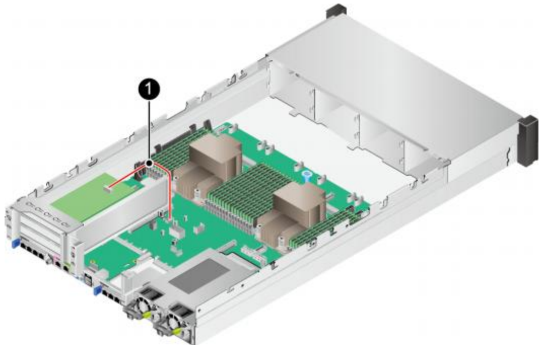
图 3-15 NC-SI 连线
