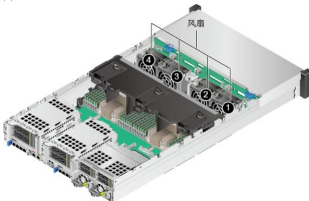
图 2-45 风扇位置图
