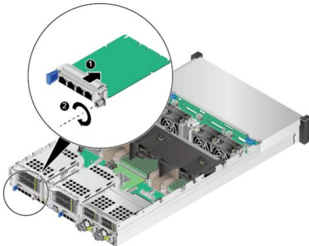
图 5-79 安装灵活 IO 卡
