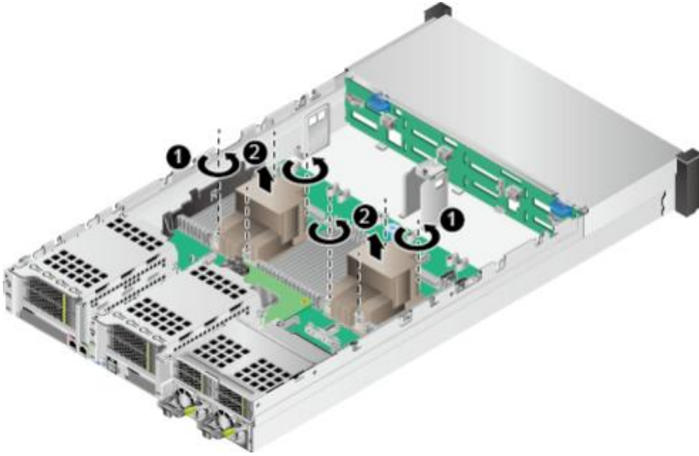
图 5-98 拆卸 CPU 散热器
