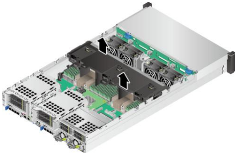
图 5-37 拆卸导风罩
