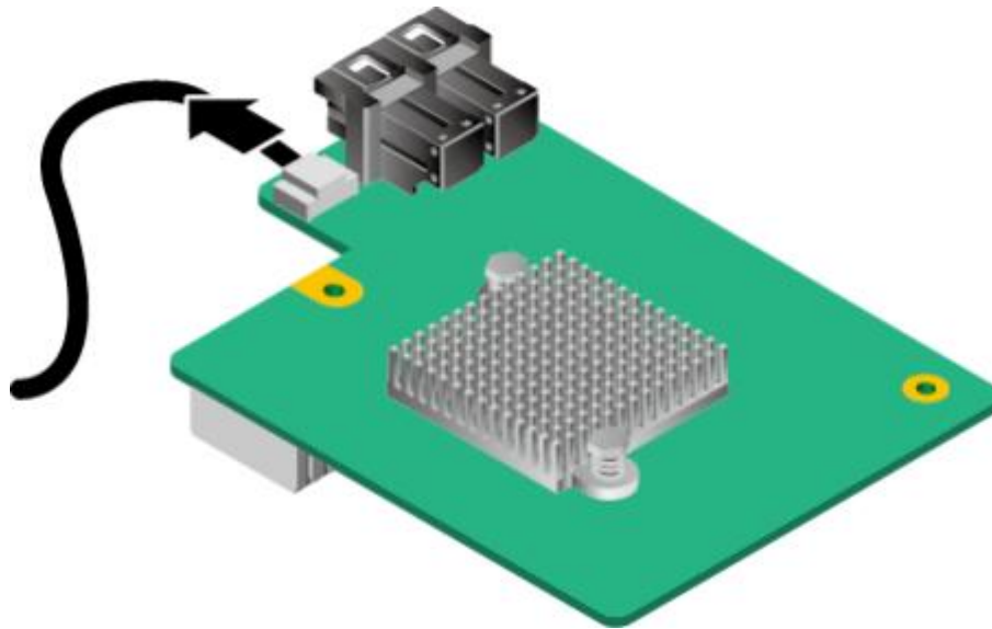
图 5-67 拔出超级电容线缆
