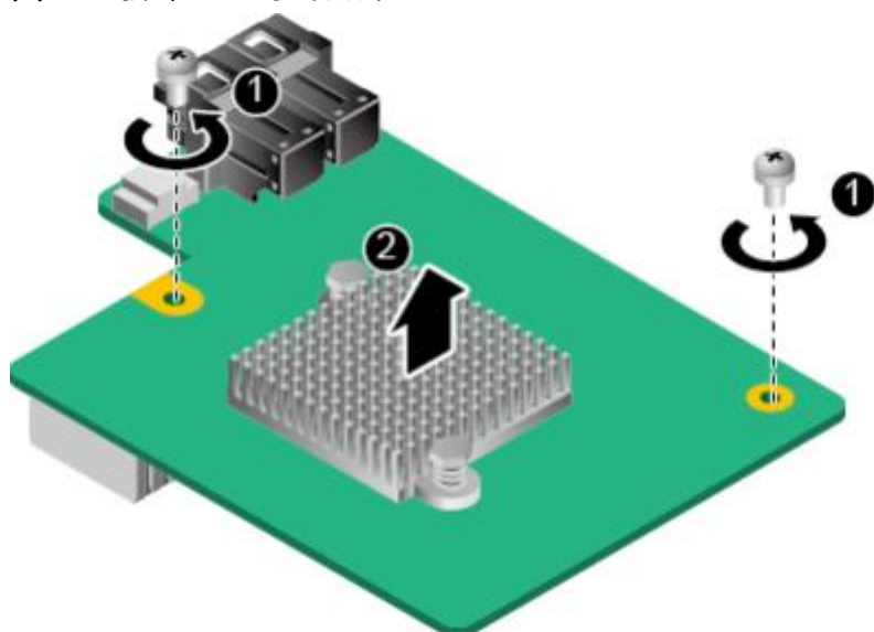
图 5-64 拆卸 RAID 控制扣卡
