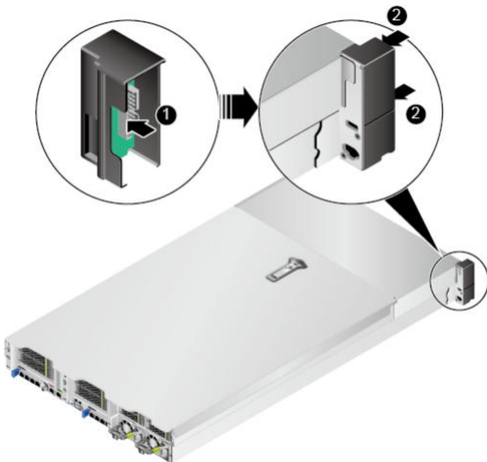
图 5-93 安装左挂耳板
