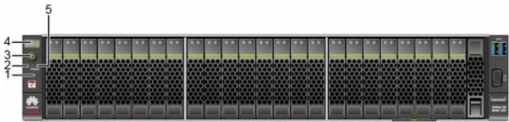
图 2-9 24x2.5 SAS/SATA 硬盘直通配置前面板指示灯和按钮
