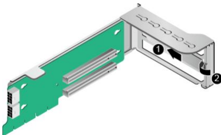
图 5-57 安装空闲挡板
