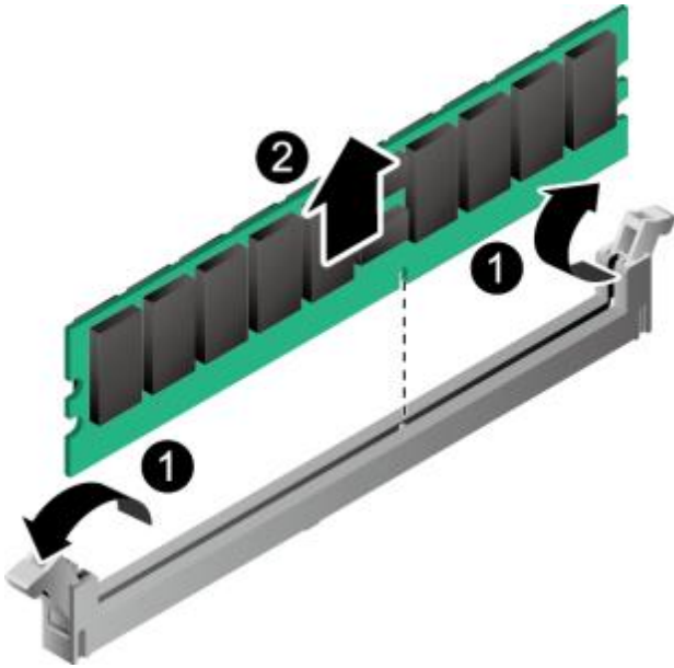
图 5-73 拆卸 DIMM
