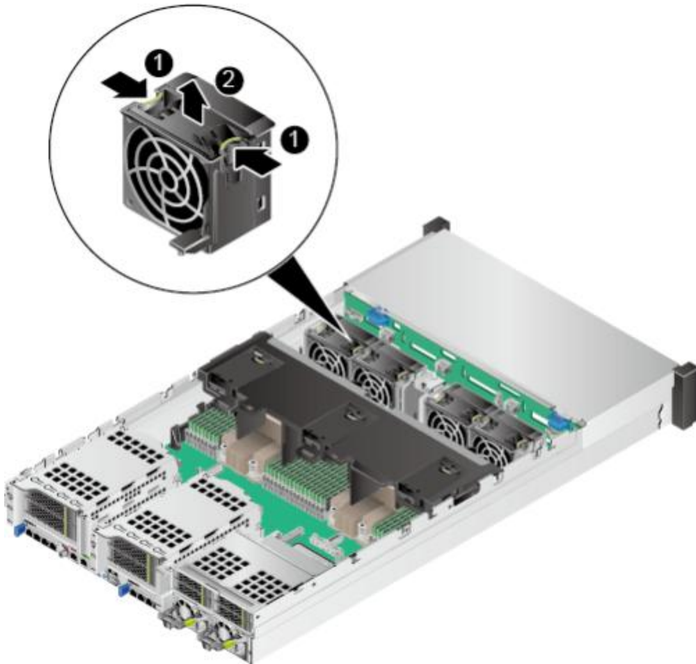
图 5-40 拆卸风扇模块
