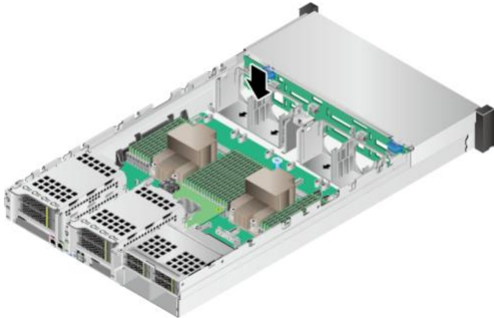
图 5-110 安装风扇支架
