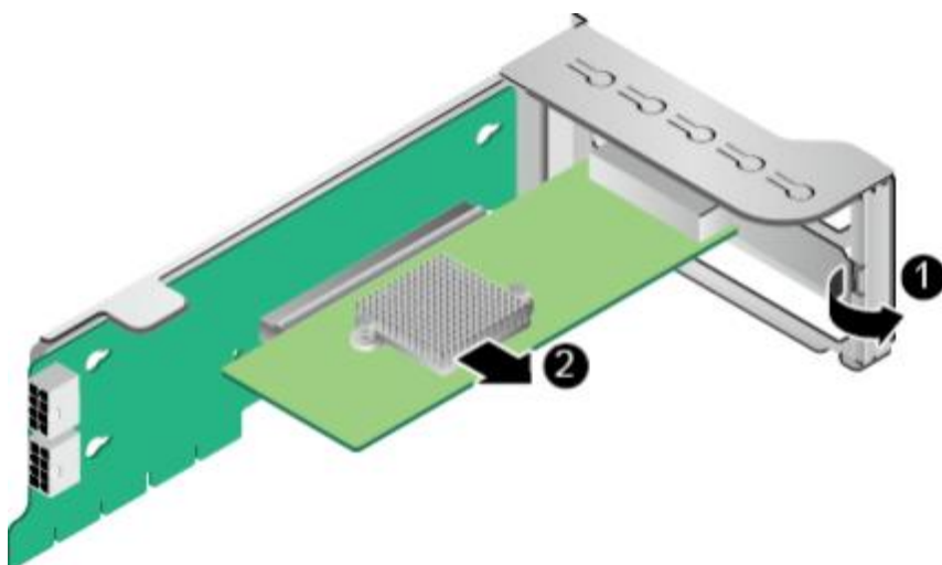
图 5-56 拆卸 Riser 模组上的 PCIe 卡
