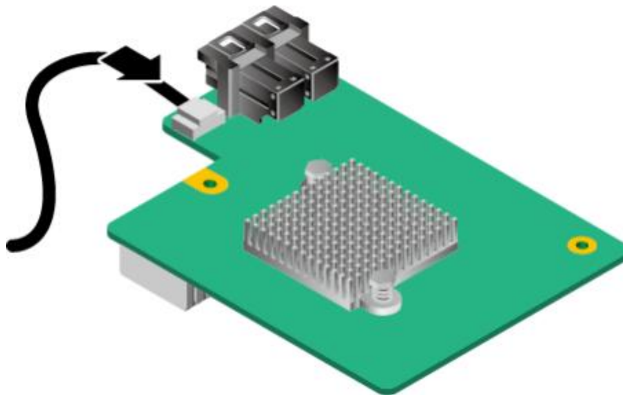
图 5-72 连接超级电容线缆
