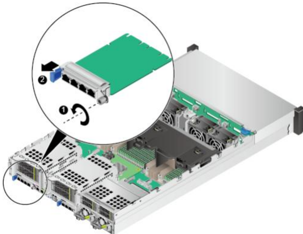
图 5-76 拆卸灵活 IO 卡
