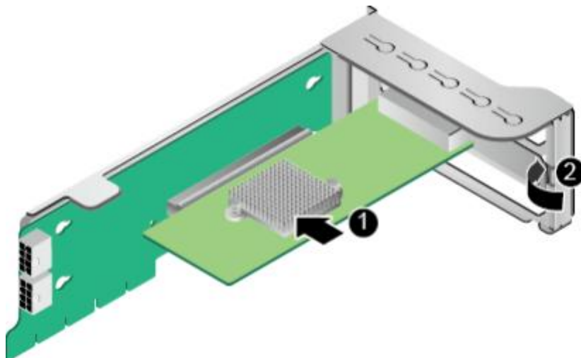
图 5-59 安装 Riser 模组上的 PCIe 卡
