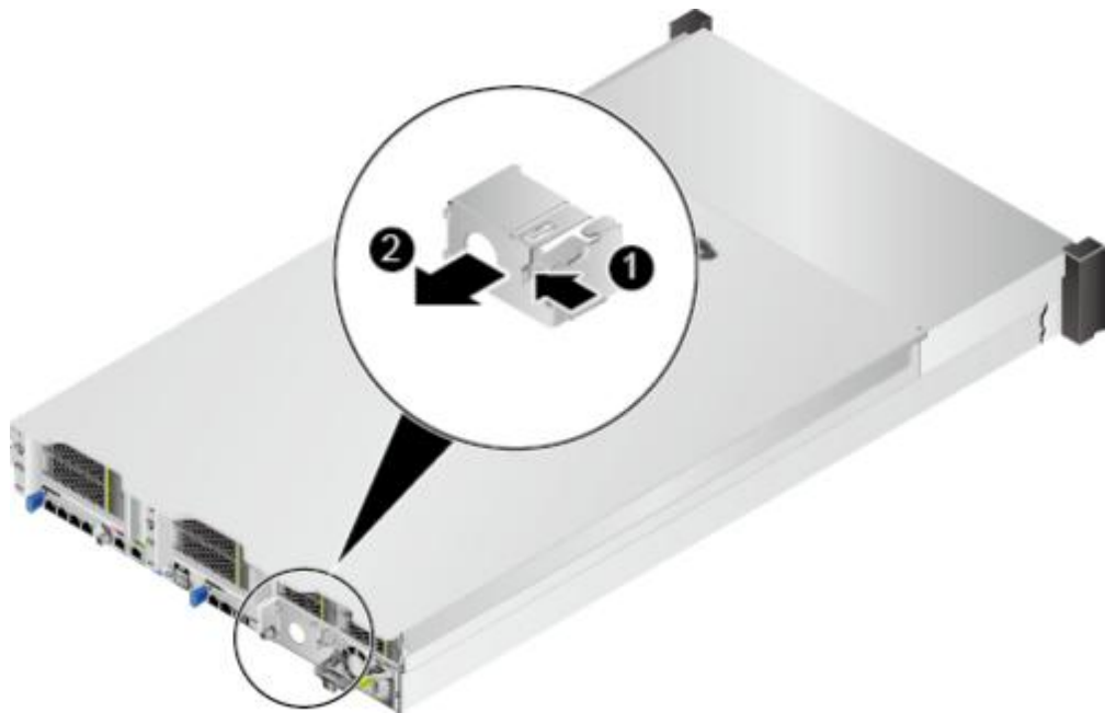
图 5-23 拆卸电源空闲挡板
