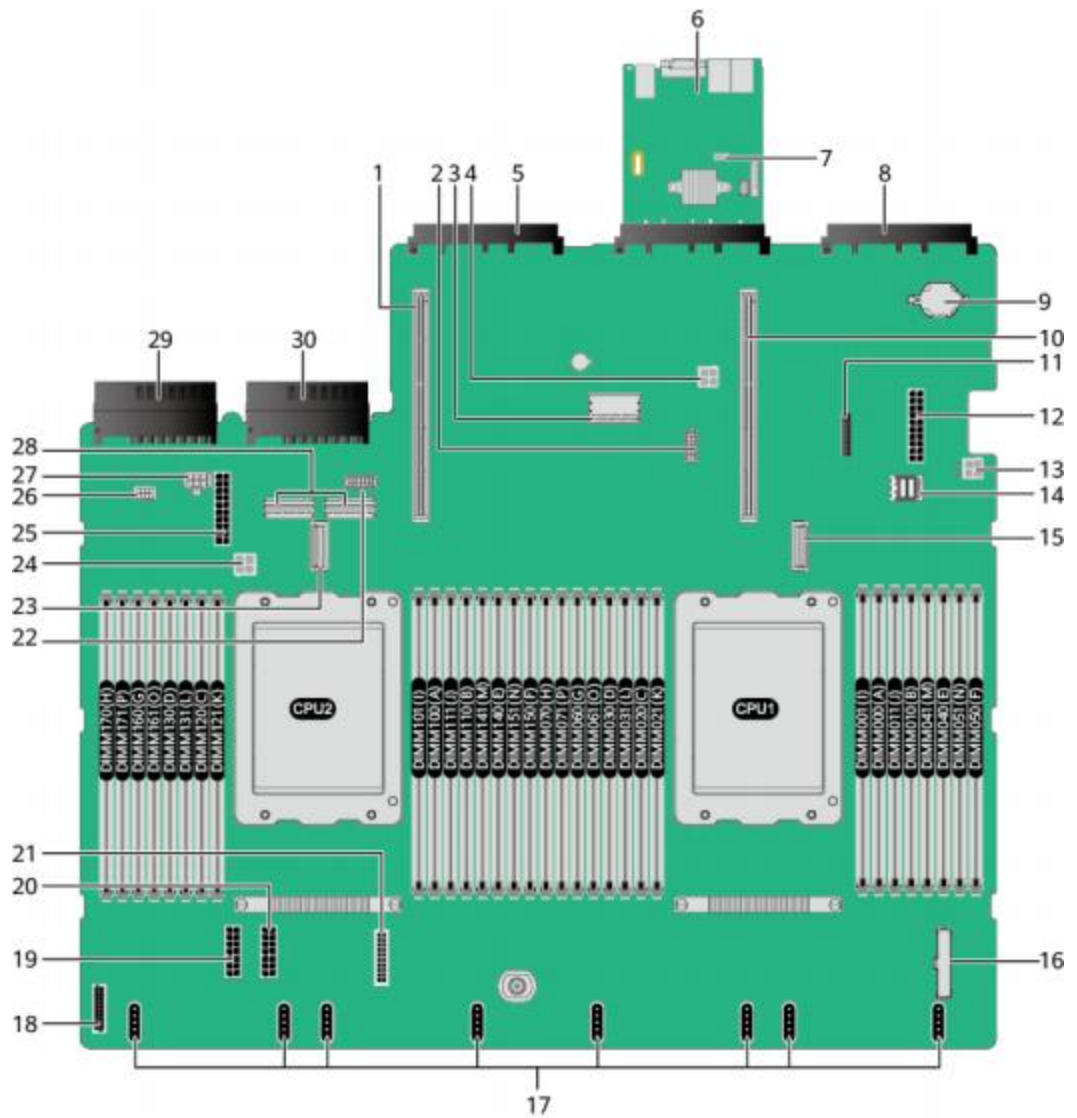
图 2-33 主板和 iBMC 插卡接口(配置鲲鹏 920 7260 或 5250 处理器)
