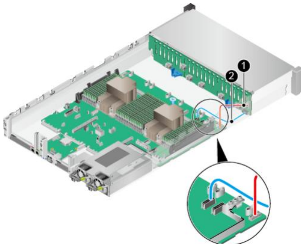
图 3-27 前置硬盘背板的电源线和低速信号线
