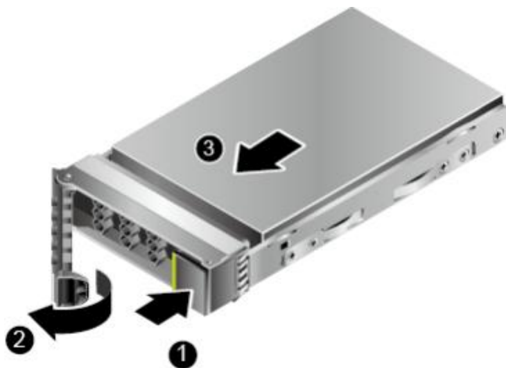
图 5-17 拆卸硬盘
