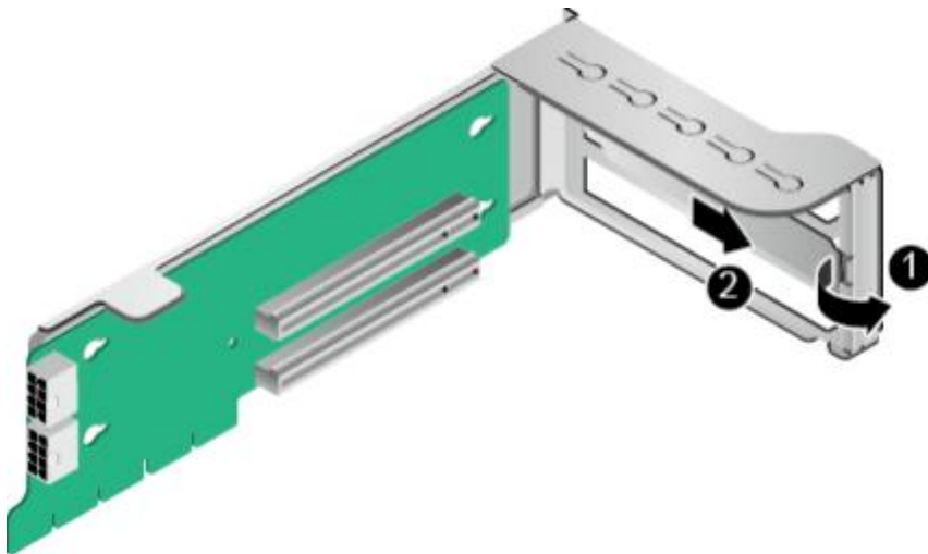
图 5-58 拆卸 PCIe 空闲挡板
