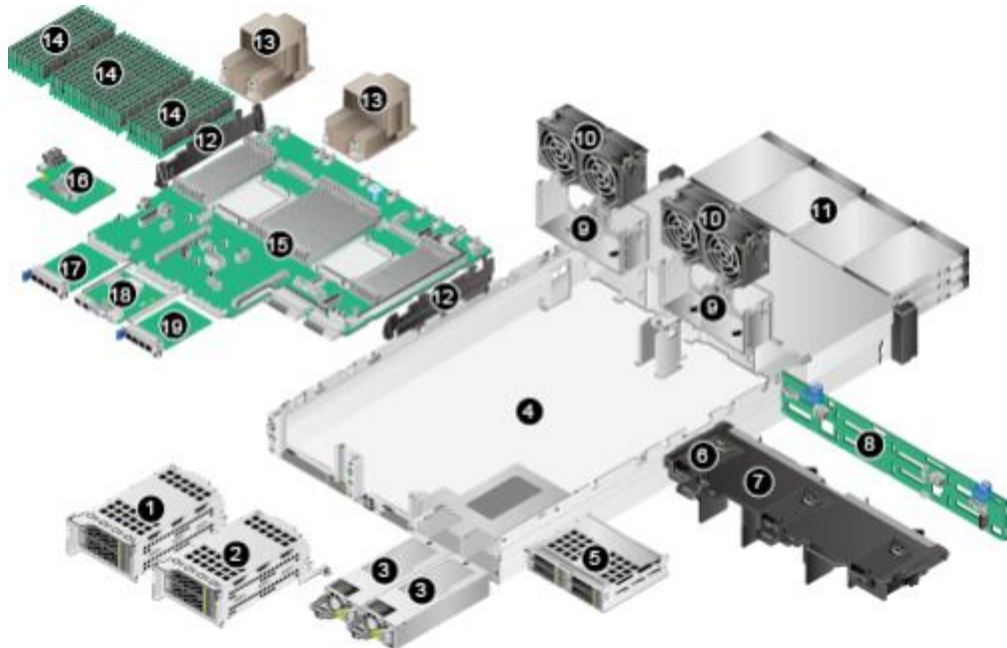
图 1-1 部件(配置鲲鹏 920 7260 或 5250 处理器)
