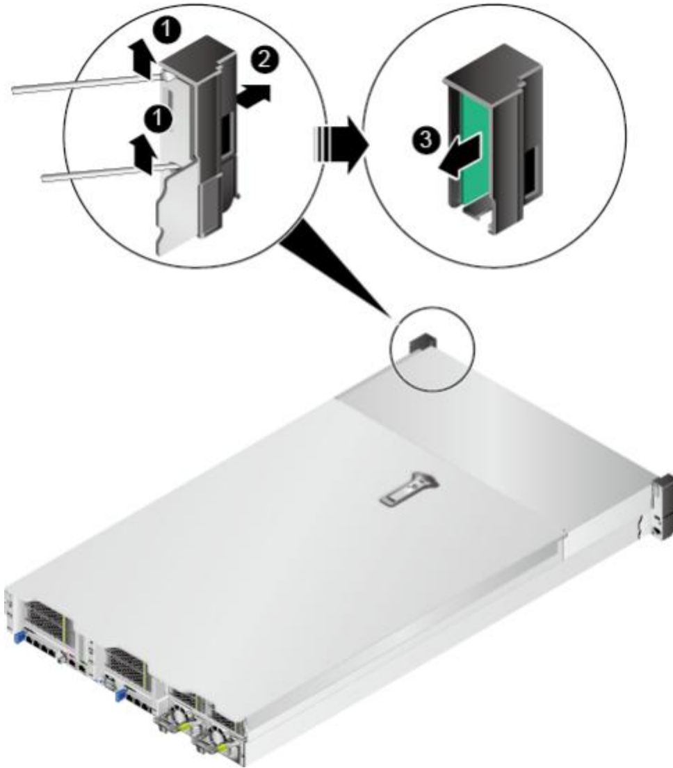
图 5-94 拆卸右挂耳板
