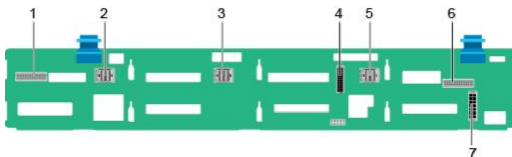
图 2-24 12x3.5 英寸硬盘直通背板( Part No.: 03025VYU )
