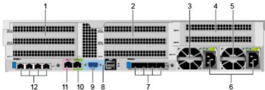
图 2-11 后面板组件
