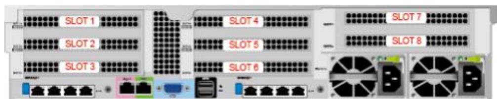
图 2-44 PCIe 插槽
