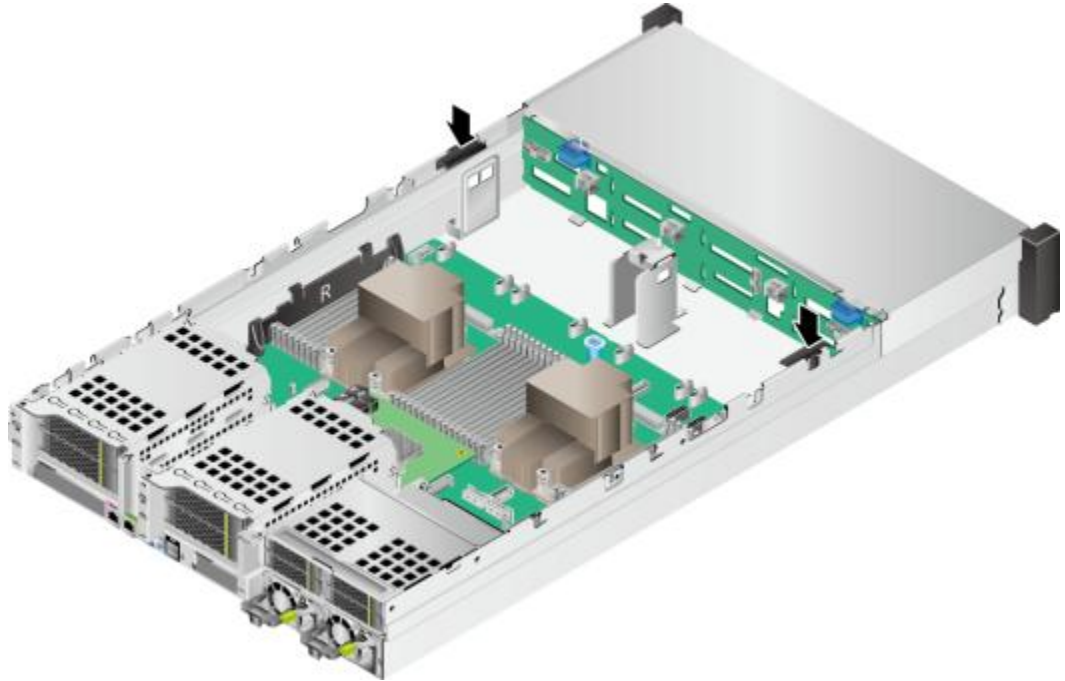
图 5-109 安装理线扣
