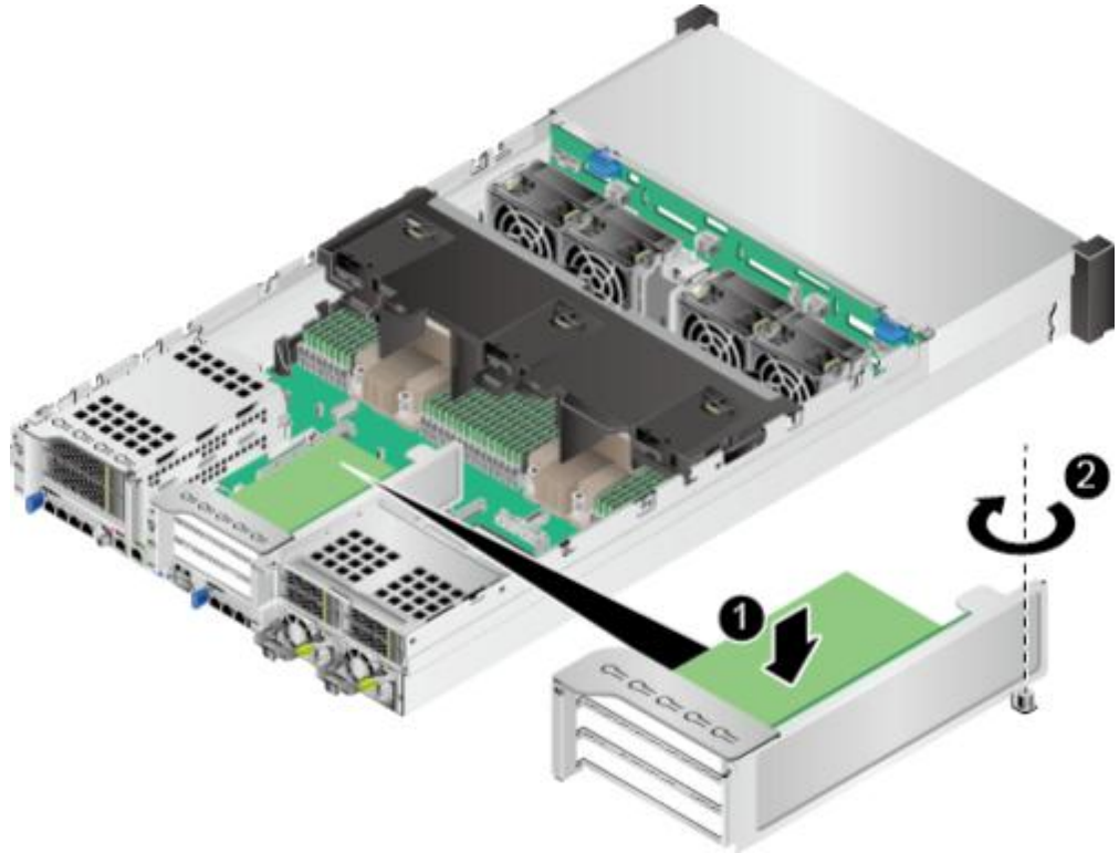
图 5-53 安装 Riser 模组 2
