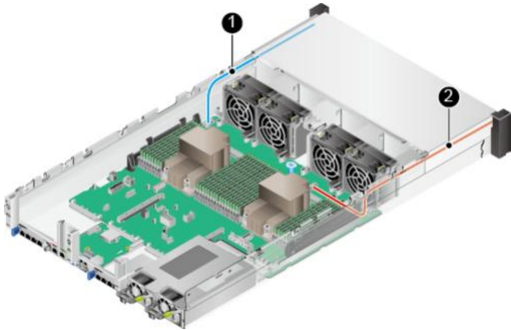
图 3-16 左右挂耳连线
