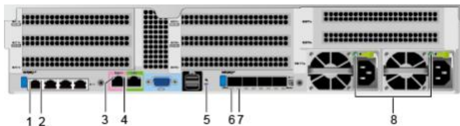
图 2-12 后面板指示灯
