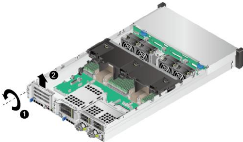
图 5-49 拆卸空闲挡板(1)
