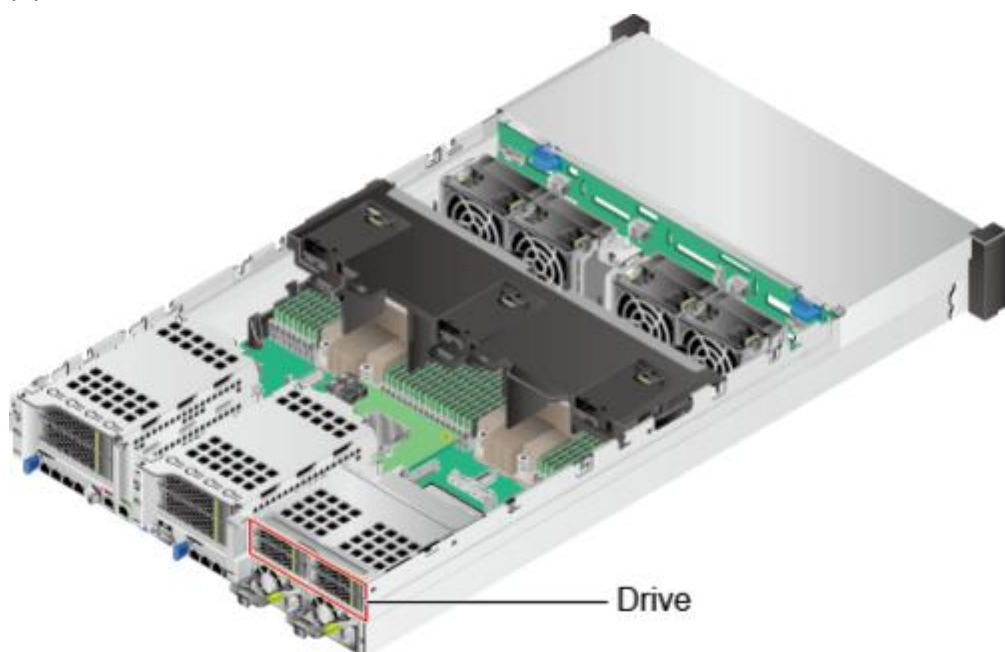
图 5-88 硬盘位置
