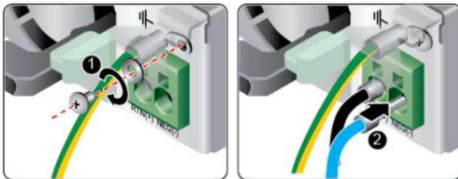
图 5-32 连接电源线缆(非 2000W 电源模块)
