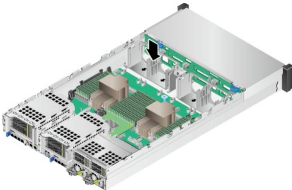
图 5-83 安装风扇支架
