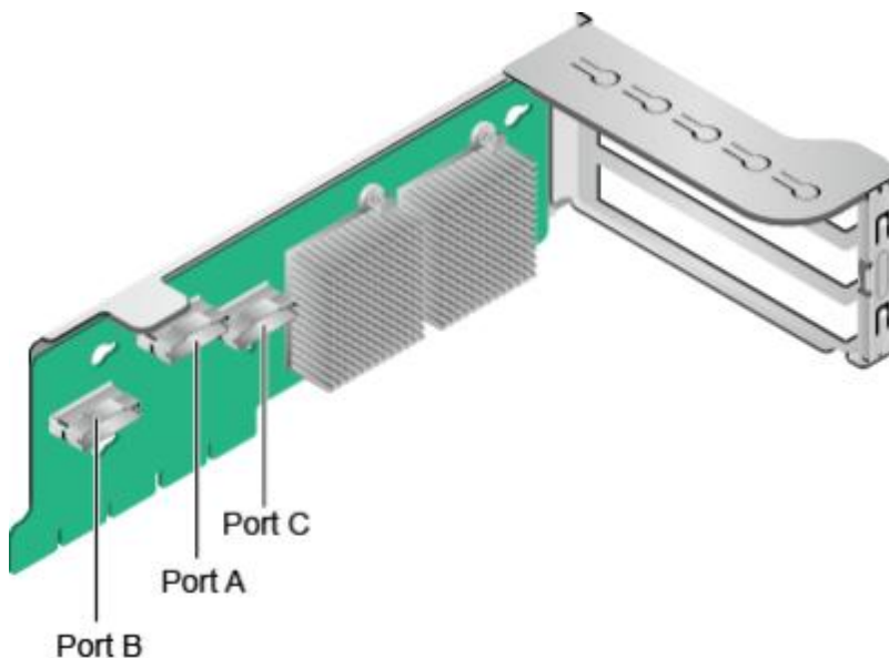
图 2-39 12NVMe 专用 Riser 卡 3 (板名: BC82PRUD)
