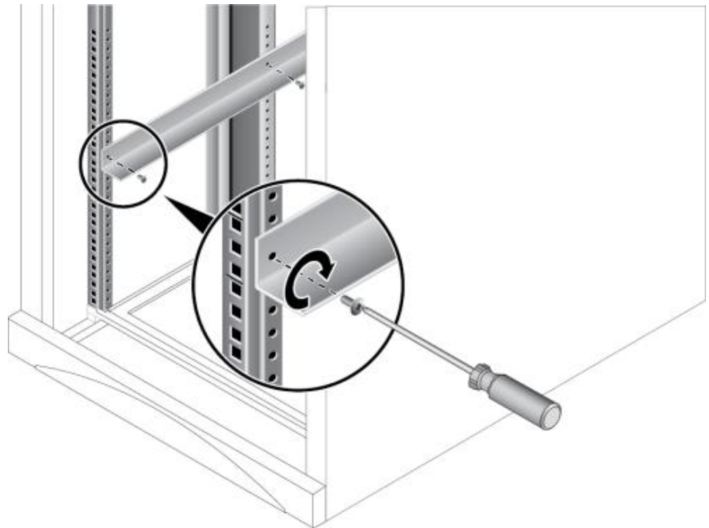
图 5-5 安装 L 型滑道
