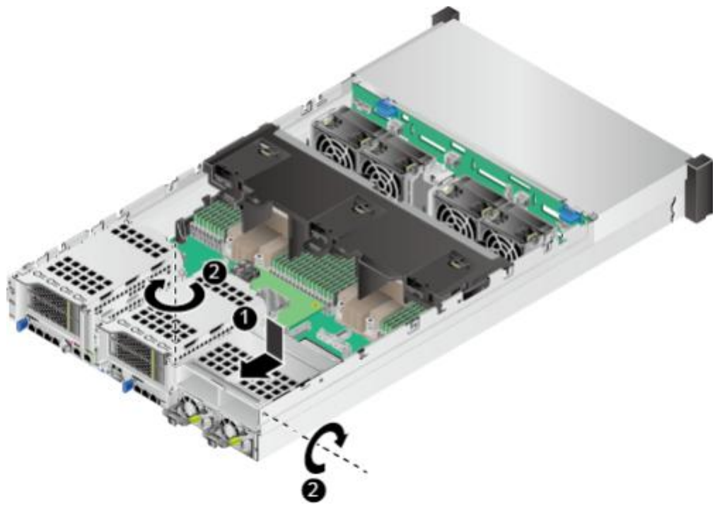
图 5-90 安装后置硬盘组件
