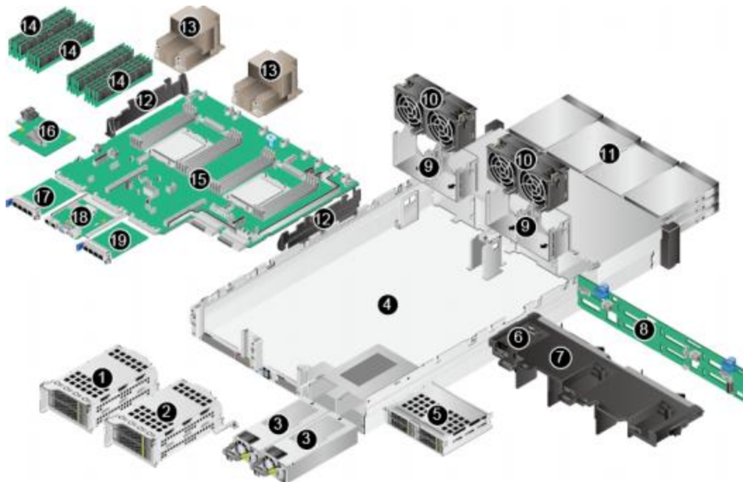
图 1-2 部件(配置鲲鹏 920 5220 或 3210 处理器)
