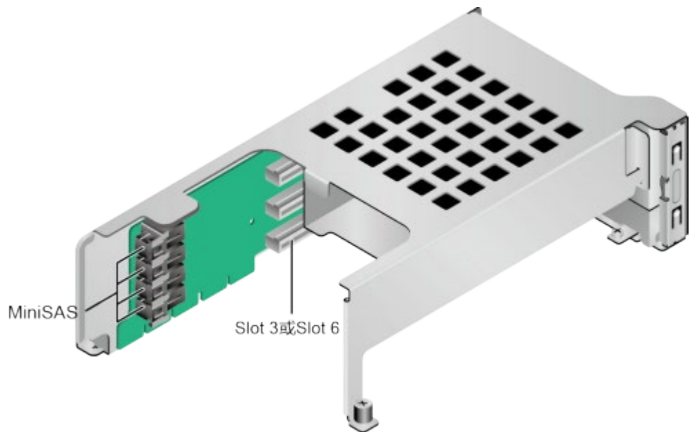
图 2-41 SAS Riser 卡 5 (板名： BC82PRNE)
