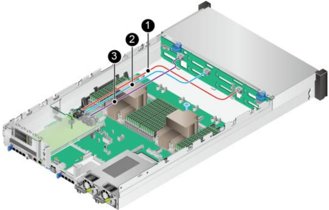
图 3-13 前置硬盘背板的 SAS 信号线
