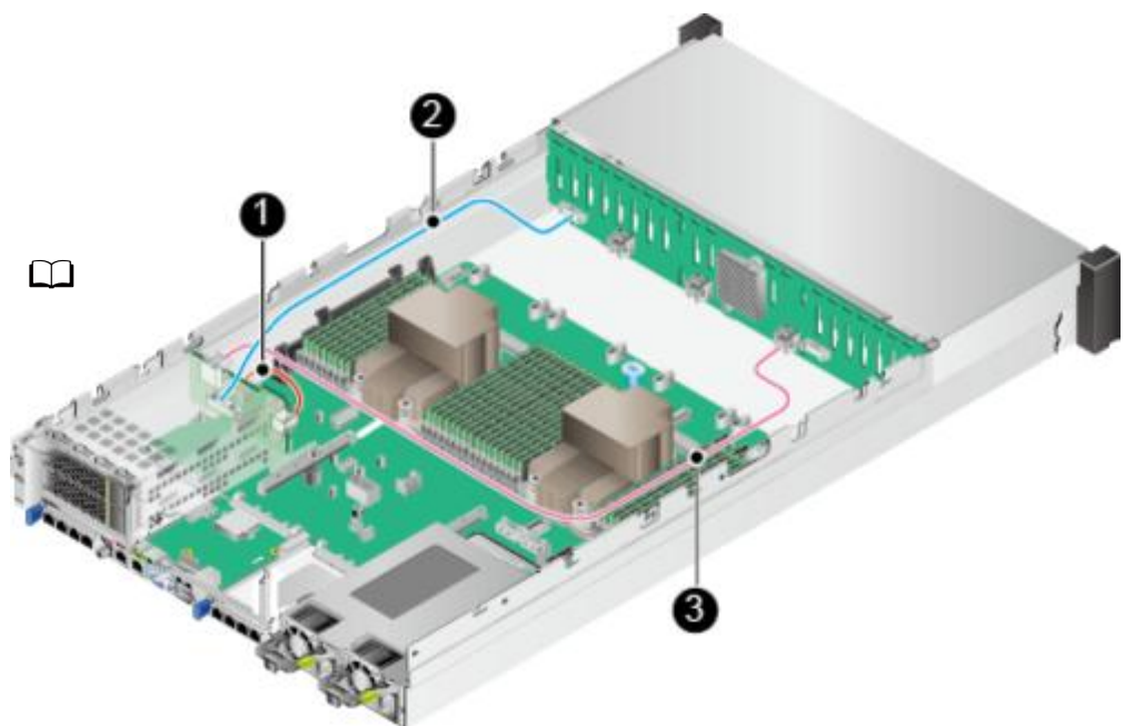
图 3-19 后置硬盘背板连线
