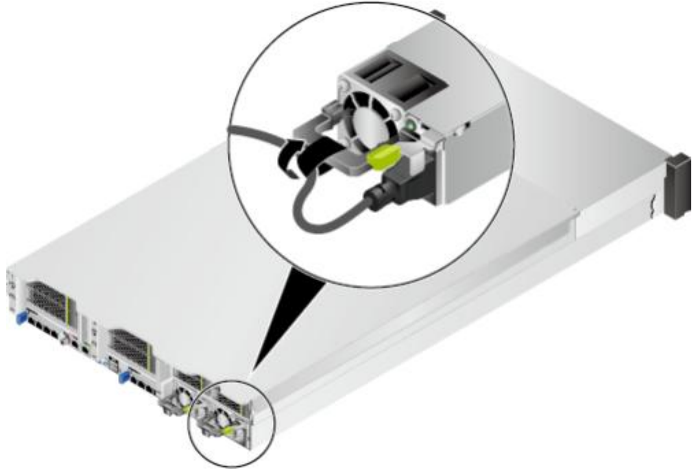
图 5-19 撕开魔术贴
