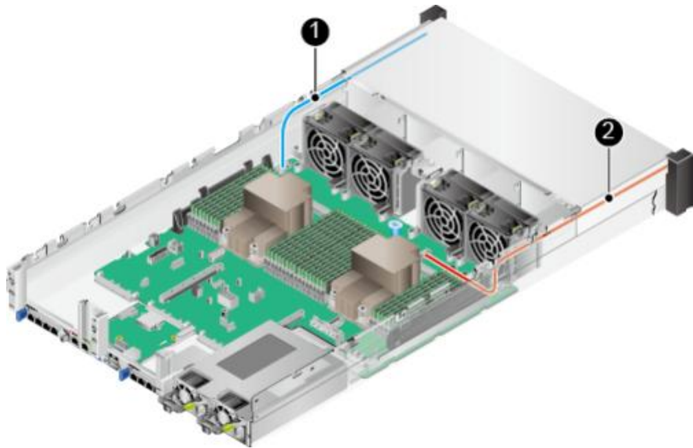
图 3-26 左右挂耳连线
