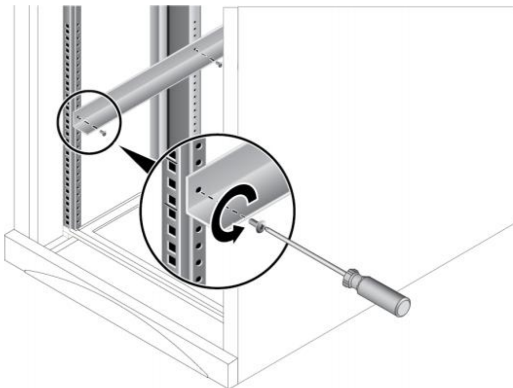
图 5-10 拆卸 L 型滑道
