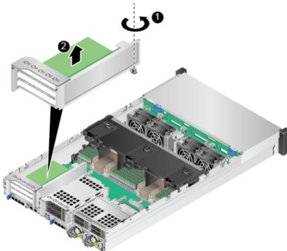
图 5-42 拆卸 Riser 模组 1
