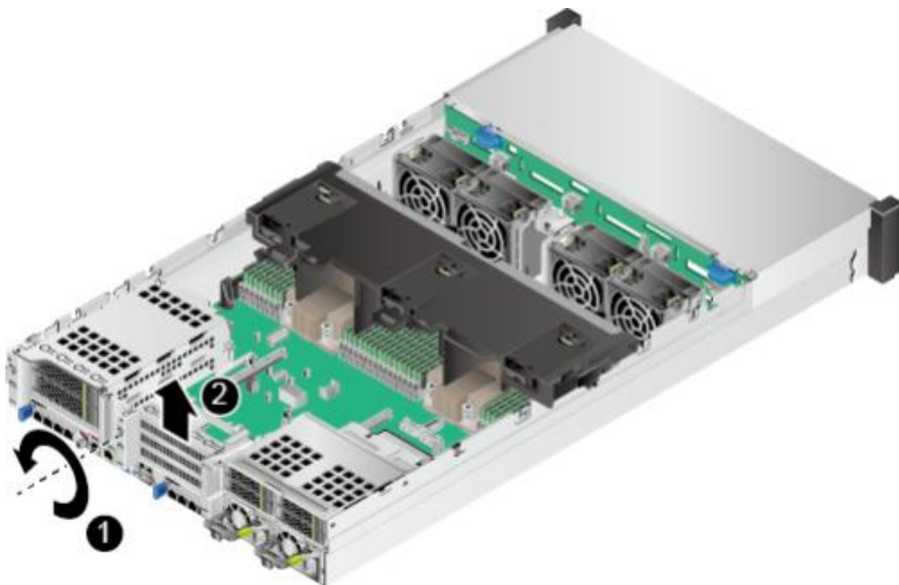
图 5-50 拆卸空闲挡板(2)
