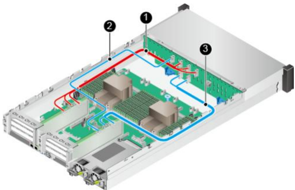
图 3-25 NVMe 硬盘扩展适配卡信号线
