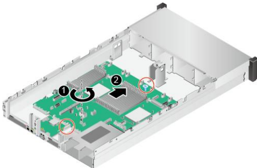
图 5-101 拆卸主板
