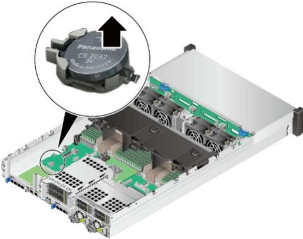
图 5-61 拆卸电池
