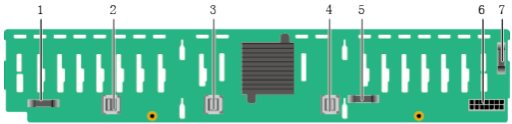
图 2-26 25x2.5 英寸硬盘背板( Part No.: 03029TDQ)
