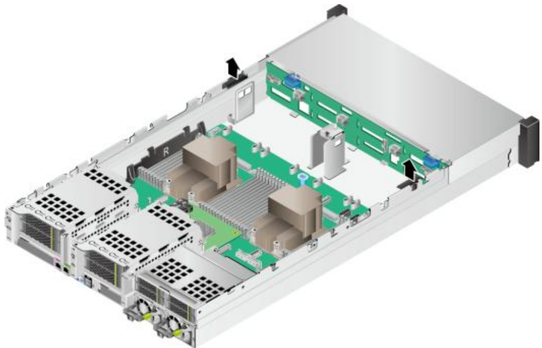
图 5-97 拆卸理线扣
