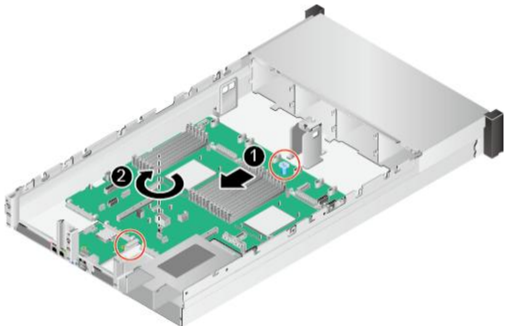
图 5-104 安装主板
