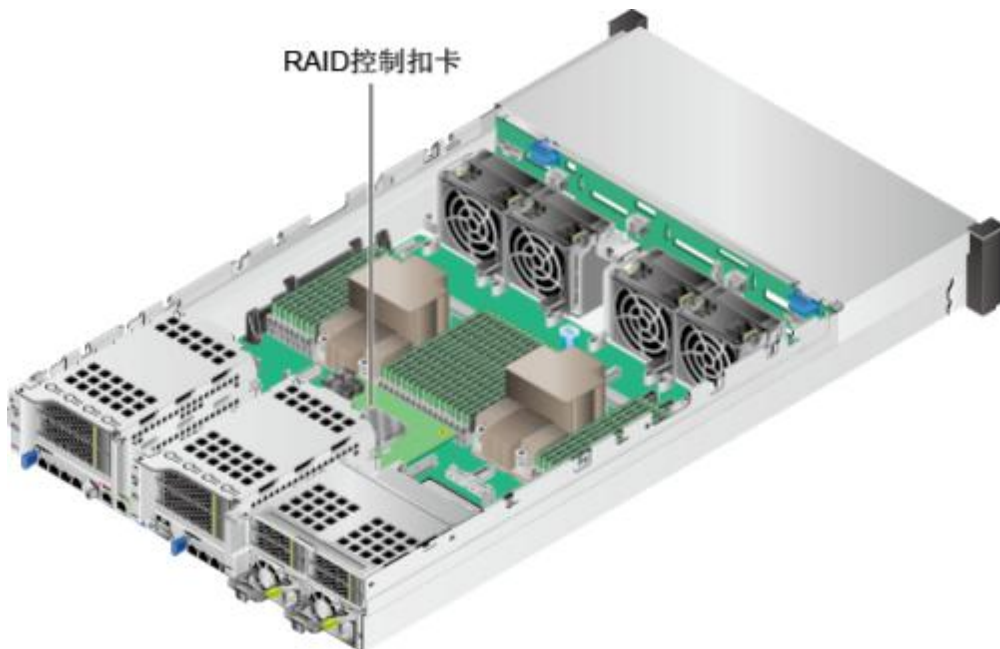
图 5-65 RAID 控制扣卡的位置
