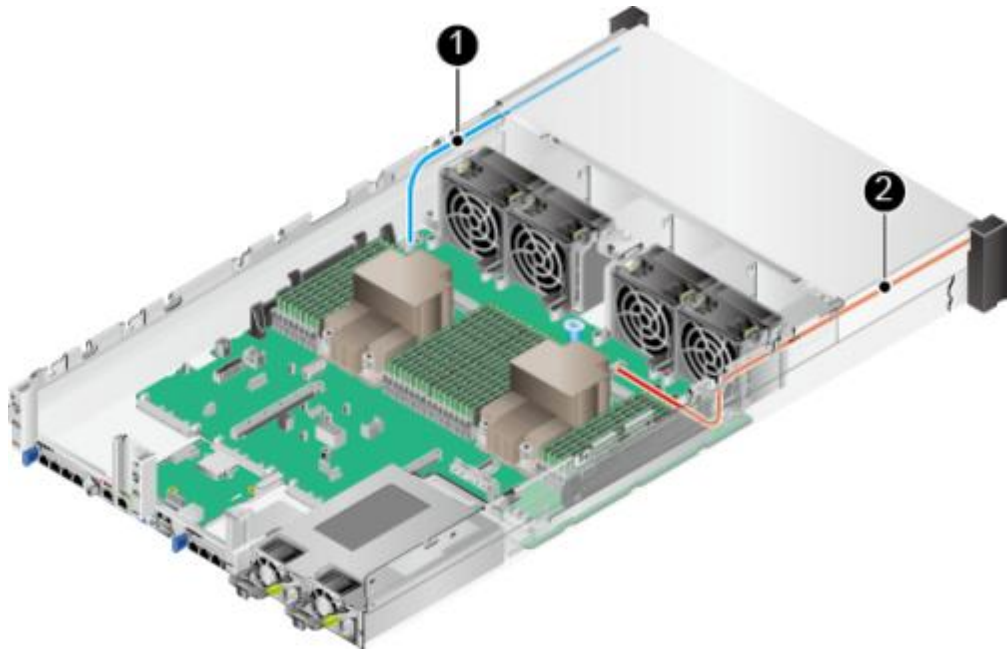
图 3-31 左右挂耳连线
