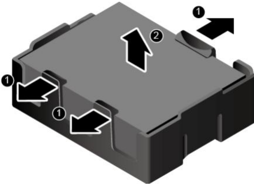
图 5-69 拆卸超级电容
