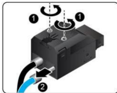
图 5-29 拆卸快插端子
