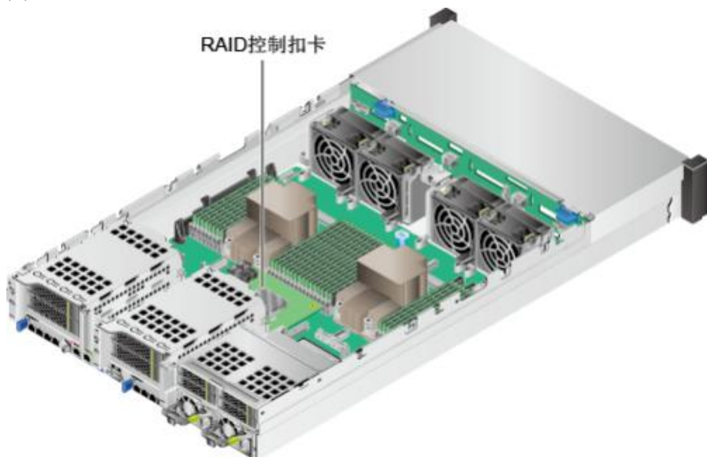
图 5-63 RAID 控制扣卡的位置
