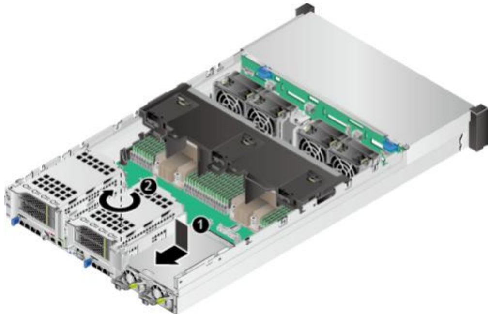
图 5-54 安装 Riser 模组 3 的下托架
