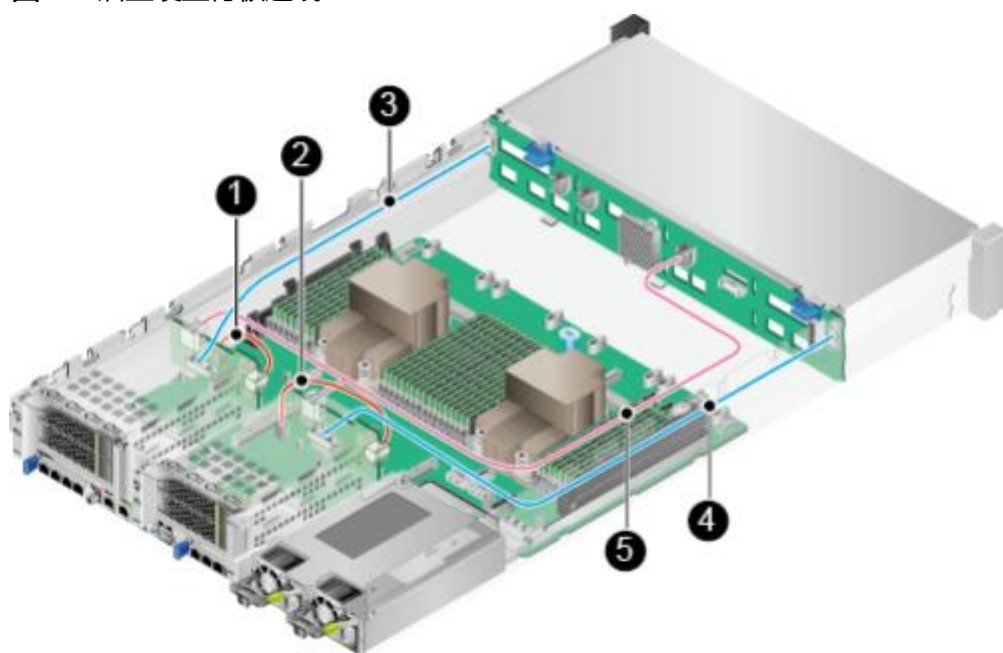
图 3-4 后置硬盘背板连线
