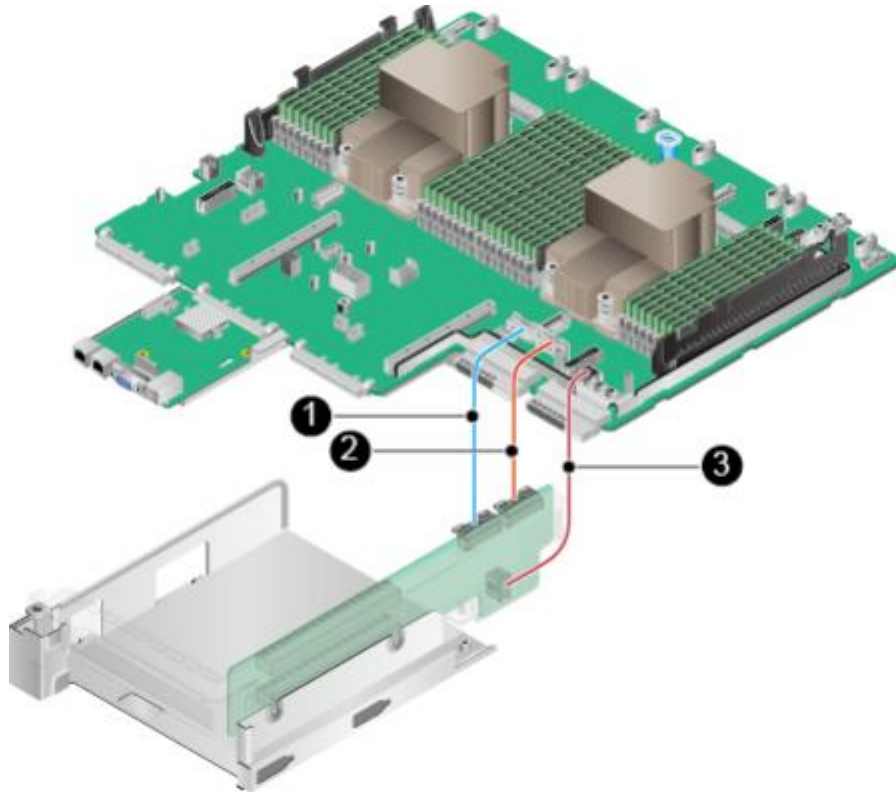
图 3-36 IO 模组 3 Riser 卡连线
