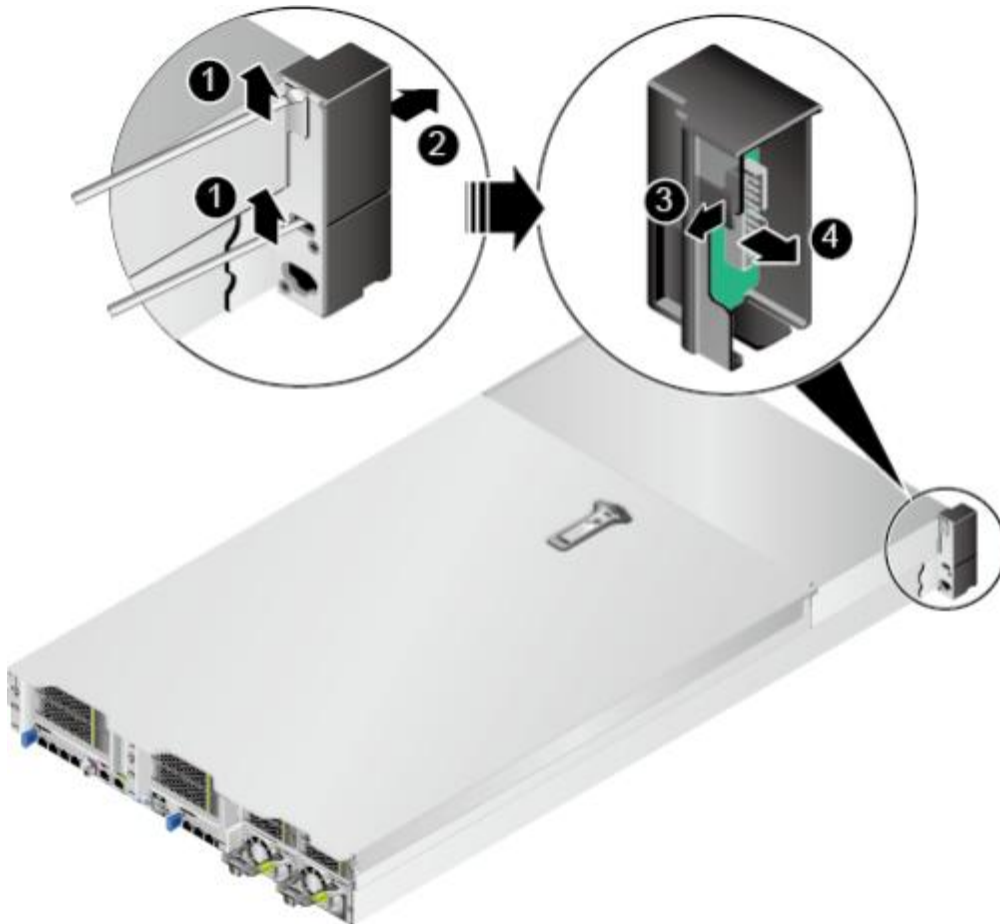
图 5-92 拆卸左挂耳板
