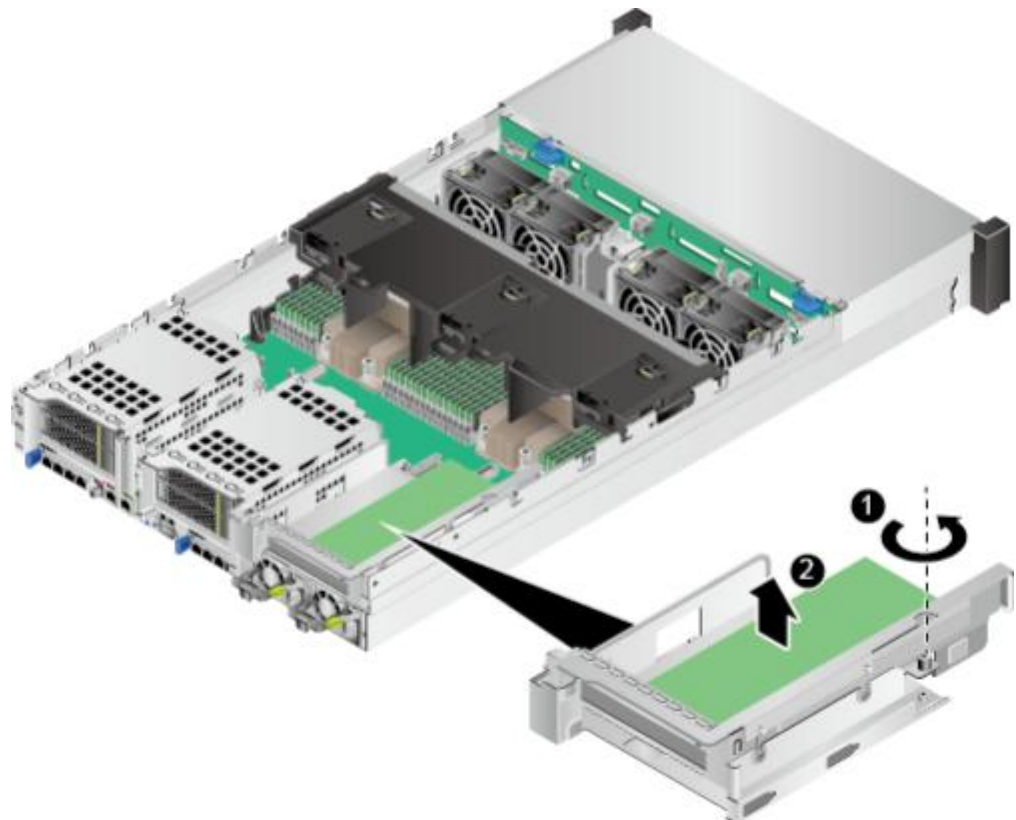
图 5-44 拆卸 Riser 模组 3 的上托架
