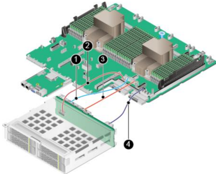
图 3-35 IO 模组 3 硬盘背板连线
