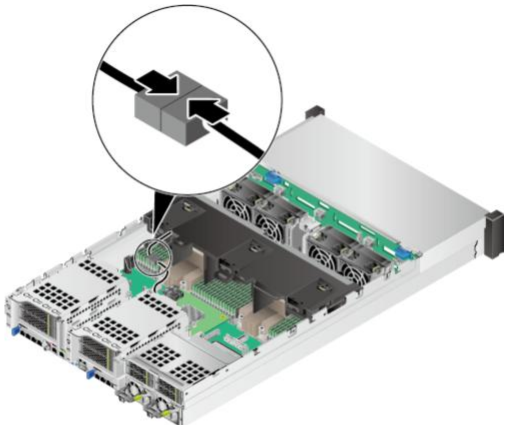
图 5-39 连接超级电容线缆
