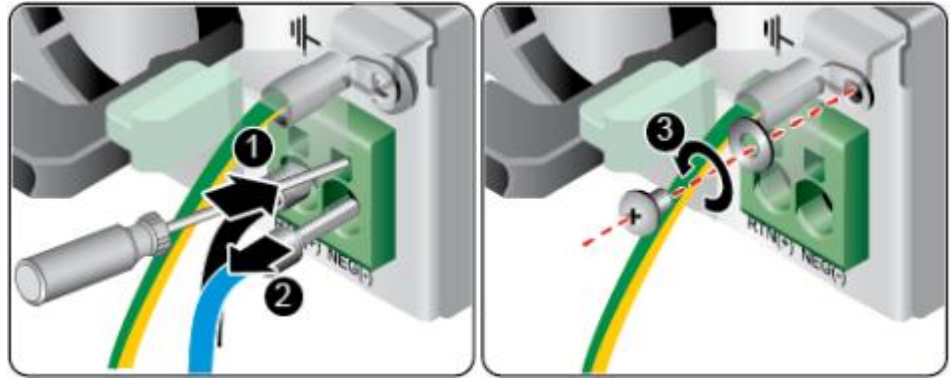
图 5-27 拔出电源线缆(非 2000W 电源模块)
