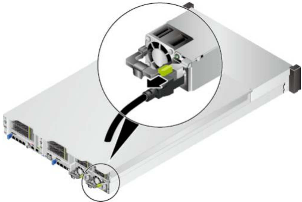
图 5-20 拔出电源线缆
