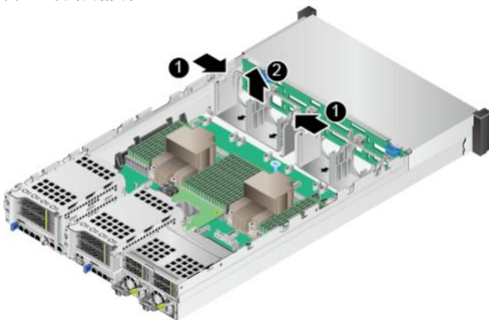
图 5-80 拆卸风扇支架
