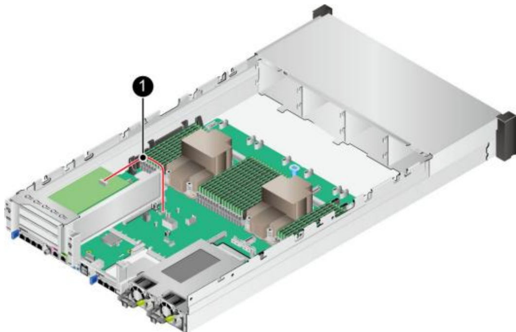
图 3-10 NC-SI 连线
