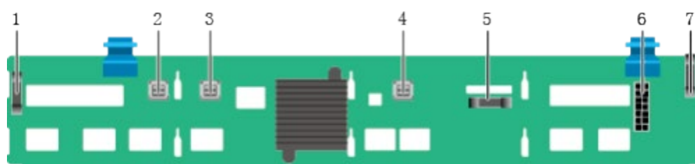
图 2-25 12x3.5 英寸硬盘 EXP 背板( Part No.: 302010155)
